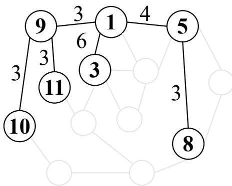
T_{\text{MonoGST}}
