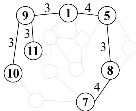
T_{\text{MonoGST+}}
