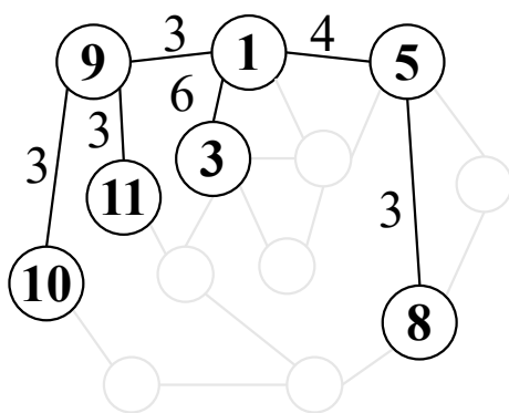
T_{\text{MonoGST}}
