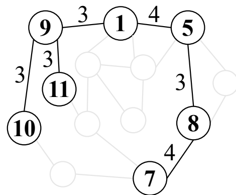
T_{\text{MonoGST+}}
