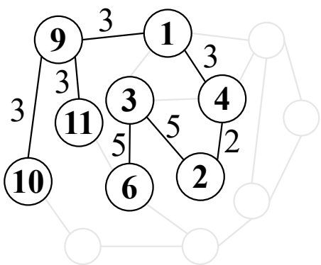
T_{\text{ImproVAPP}}
