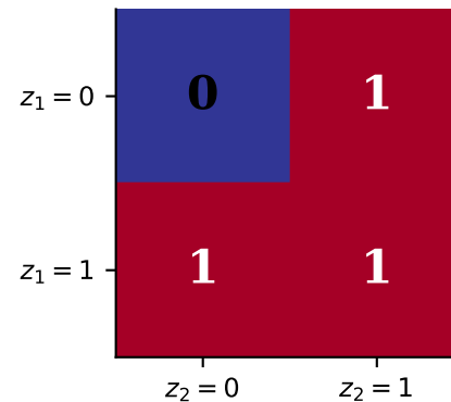
OR: z_1 \vee z_2
