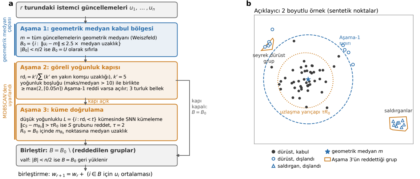
Şekil 1. Fed-MDBSCAN-G yönteminin karar yolu. (a) Aşama 1 geometrik medyan çevresinde ilk havuz B_0 'ı oluşturur; Aşama 2 küme aşamasını yalnızca göreceli yoğunluk boşluğu Aşama-1 retleriyle birlikte görüldüğünde açar; Aşama 3 düşük yoğunluklu kümeyi kümeler ve merkezi B_0 'ın geometrik medyanından \tau R_0 'dan daha uzak olan grupları reddeder. Son küme her zaman B \subseteq B_0 koşulunu sağlar. (b) Kullanılan aşama fonksiyonlarının sentetik noktalar üzerinde ürettiği açıklayıcı iki boyutlu örnek (deney verisi değildir). Aşama 1 saldırganları dokuz düğümle birlikte dışlar; Aşama 3'ün reddettiği iki grubun tamamı B_0 dışında kaldığından küme aşaması kabul kümesini değiştirmez. Bölüm VIII, kayıtlı kontrol noktalarında her aşamanın ne sıklıkla çalıştığını raporlar.
