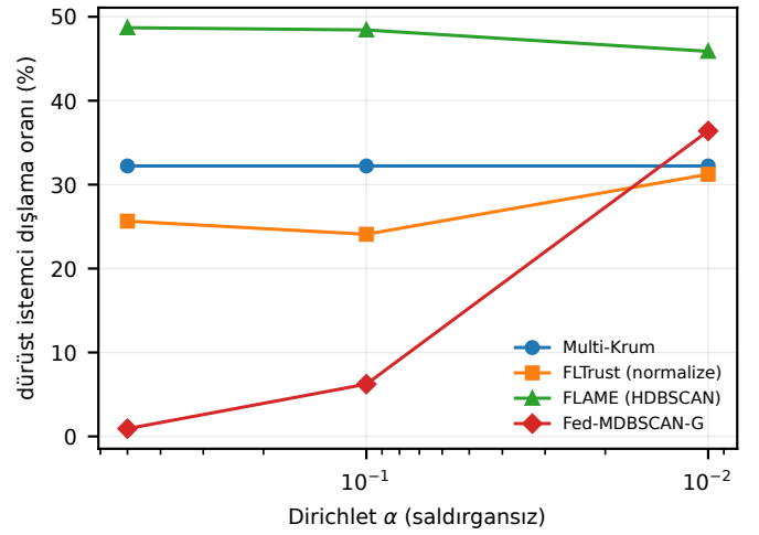
Şekil 2. Mevcut veri kümesi hücreleri üzerinden ortalananmış saldırgansız dışlama. Kapsam yoğunlaşma değerine ve yöntemine göre değişir. FLTrust sıfır ağırlıklı gönderimleri sayar. FLAME sınırına her turda ulaşılması gerekmez; doğrudan boyutlar Tablo V içindedir.
