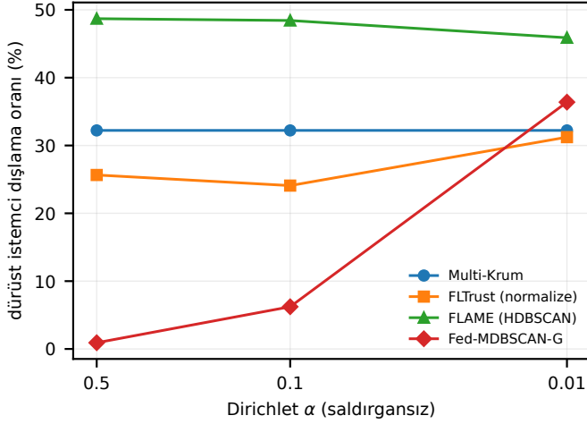
Şekil 2. Mevcut veri kümesi hücreleri üzerinden ortalananmış saldırıgansız dışlama. Kapsam yoğunlaşma değerine ve yöntemine göre değişir. FLTrust sıfır ağırlıklı gönderimleri sayar. FLAME sınırına her turda ulaşılması gerekmez; doğrudan boyutlar Tablo V içindedir.
