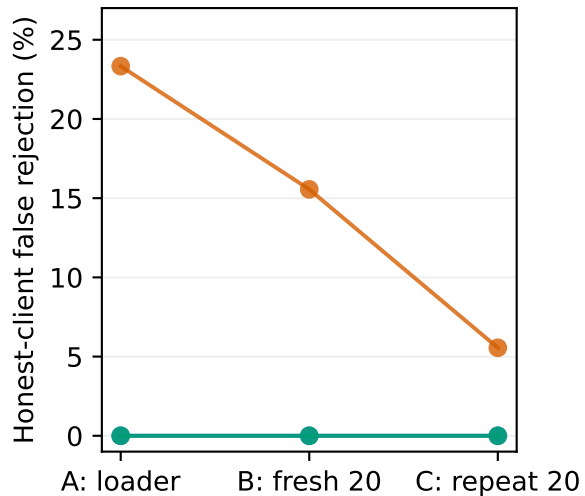
MNIST
