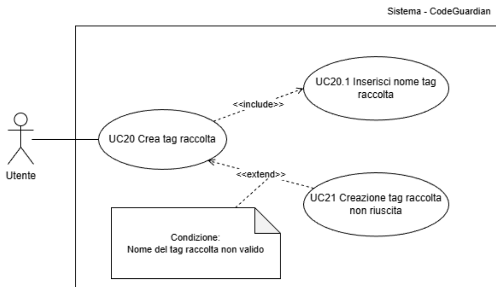
Figura 30: UC20 - Crea tag G raccolta G
