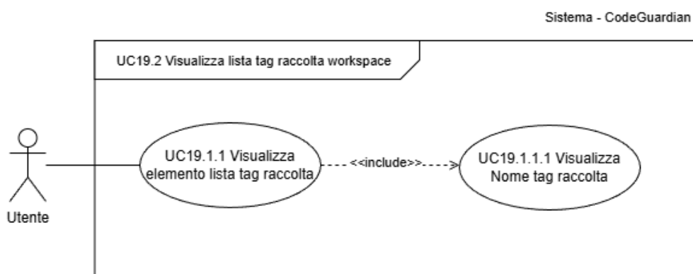
Figura 29: UC19.2 - Visualizza lista tag G raccolta G workspace
