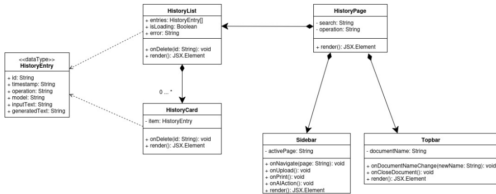
Figura 6: Diagramma UML dei componenti della View: composizione di HistoryPage
