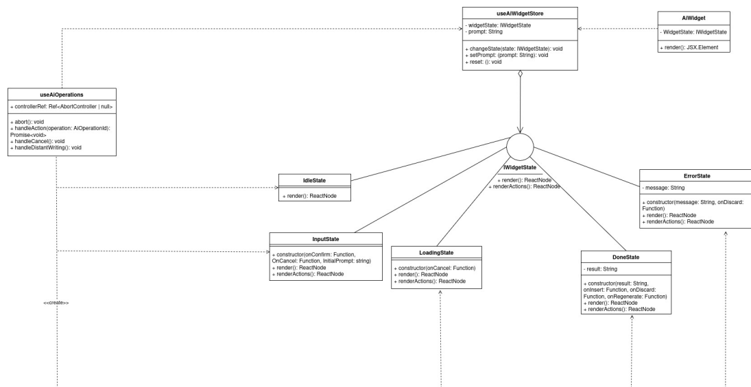
Figura 9: Diagramma delle classi del Render-Delegate State Pattern
