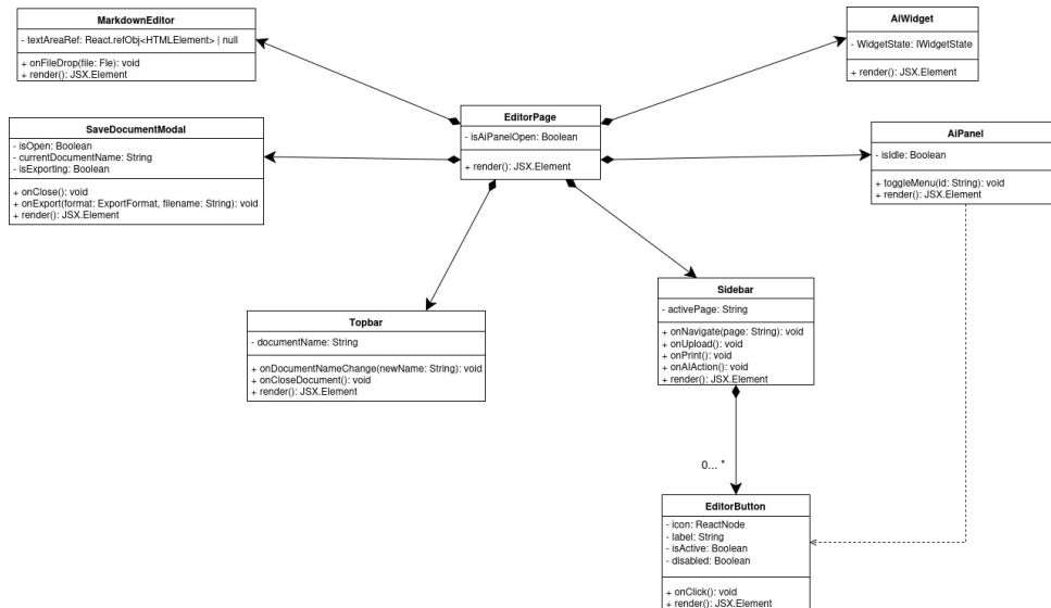
Figura 5: Diagramma UML dei componenti della View: composizione di EditorPage
