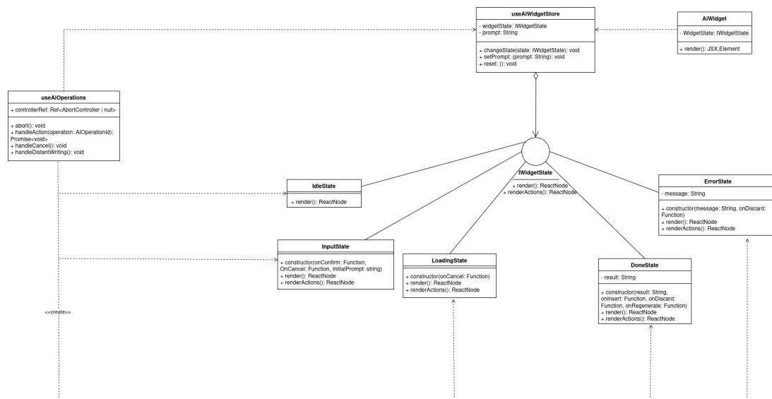
Figura 9: Diagramma delle classi del Render-Delegate State Pattern
