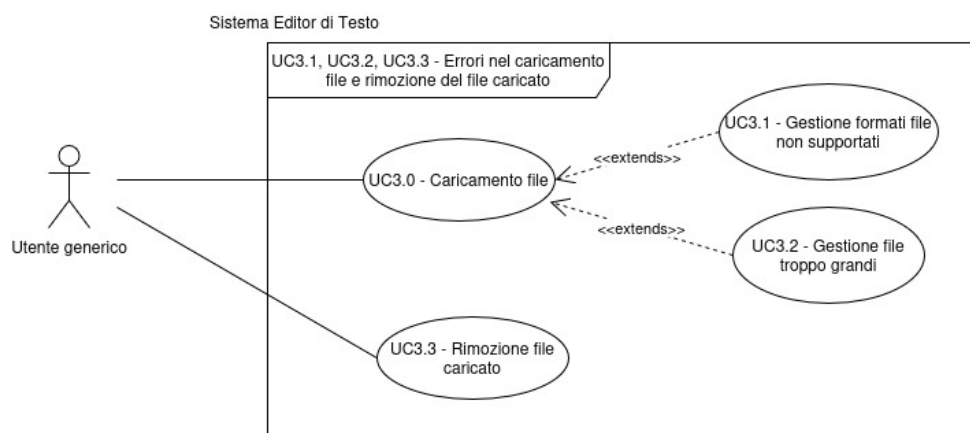
Figura 23: Diagramma dei casi d'uso UC-3.1, 3.2, 3.3
