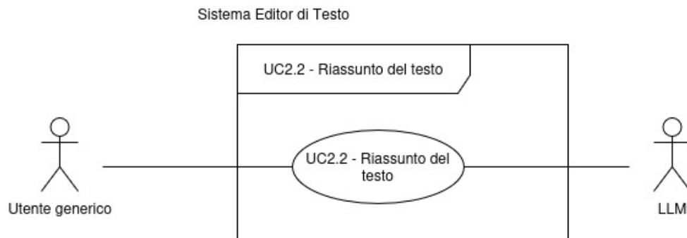
Figura 12: Diagramma dei casi d'uso UC-2.2
