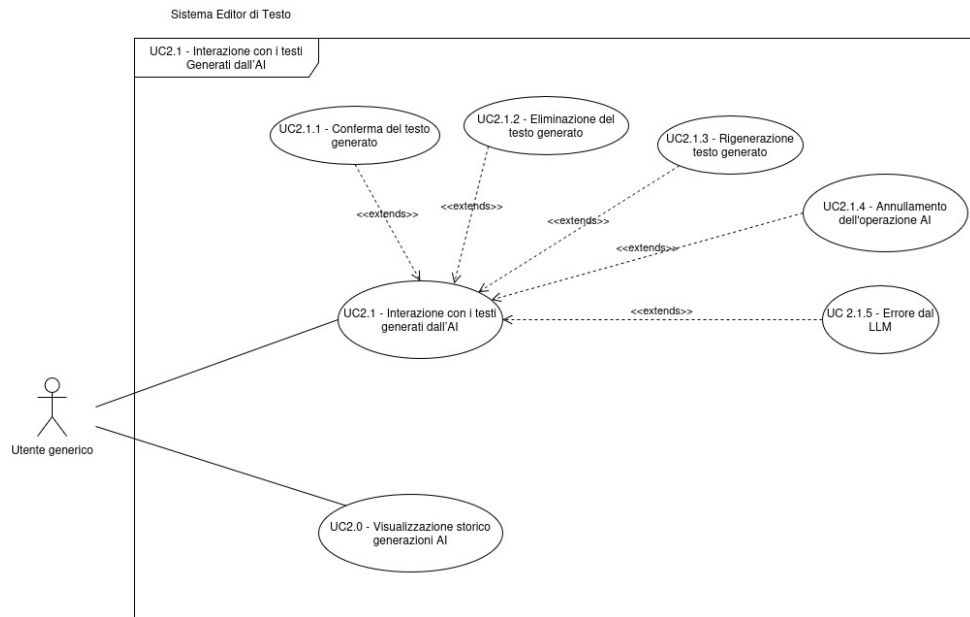
Figura 11: Diagramma dei casi d'uso UC-2.1, 2.1.*
