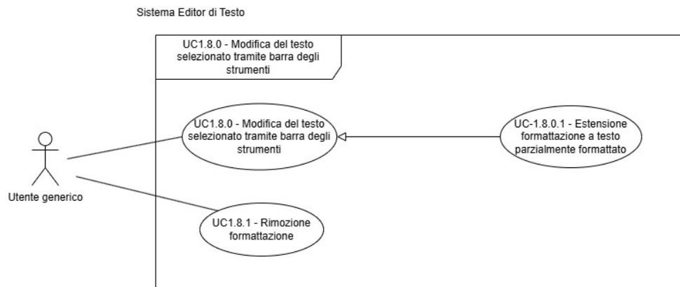
Figura 6: Diagramma dei casi d'uso UC-1.8.0, 1.8.0.1, 1.8.1
