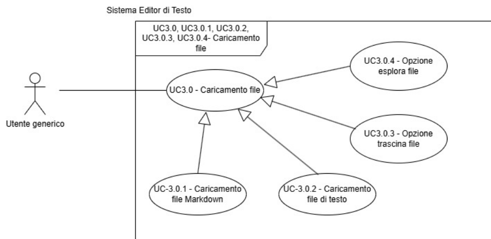
Figura 24: Diagramma dei casi d'uso UC-3.0, 3.0.*
