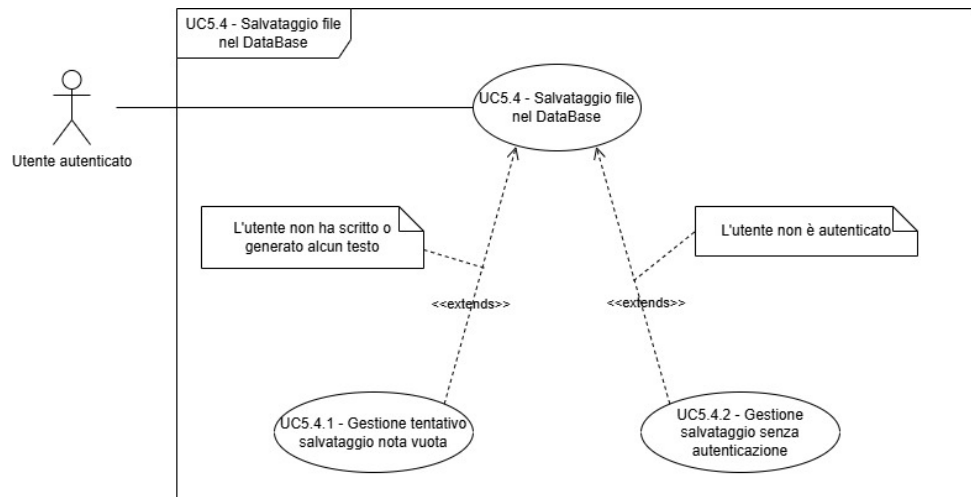
Figura 32: Diagramma dei casi d'uso UC-5.4, 5.4.1, 5.4.2
