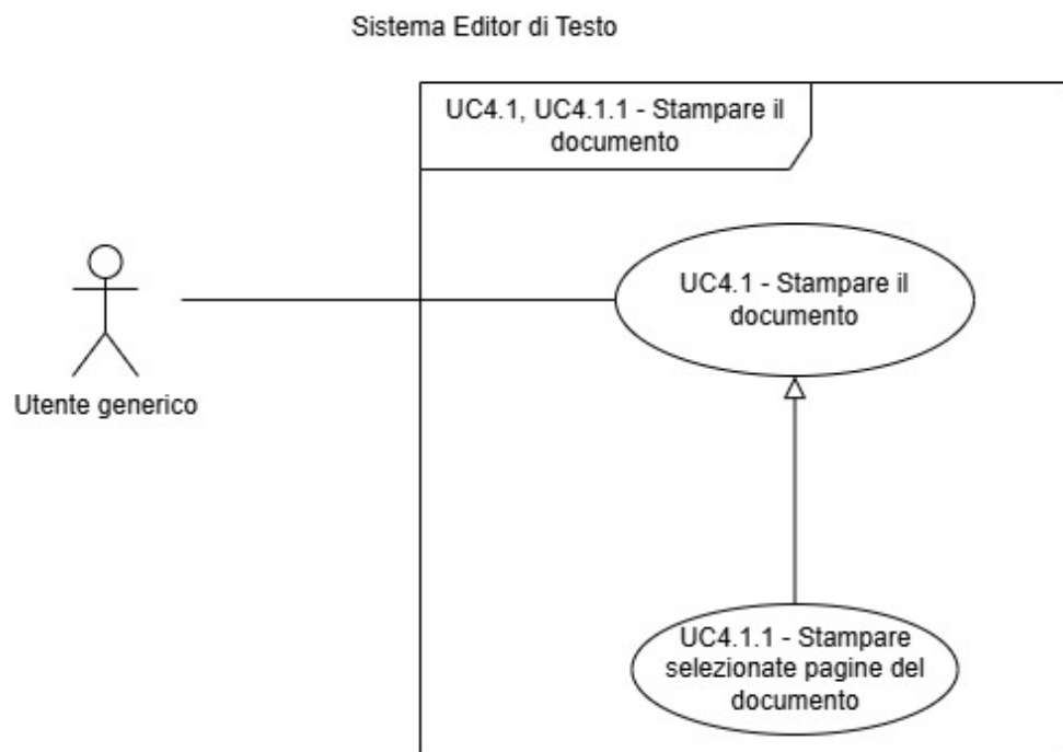
Figura 28: Diagramma dei casi d'uso UC-4.1, UC-4.1.1
