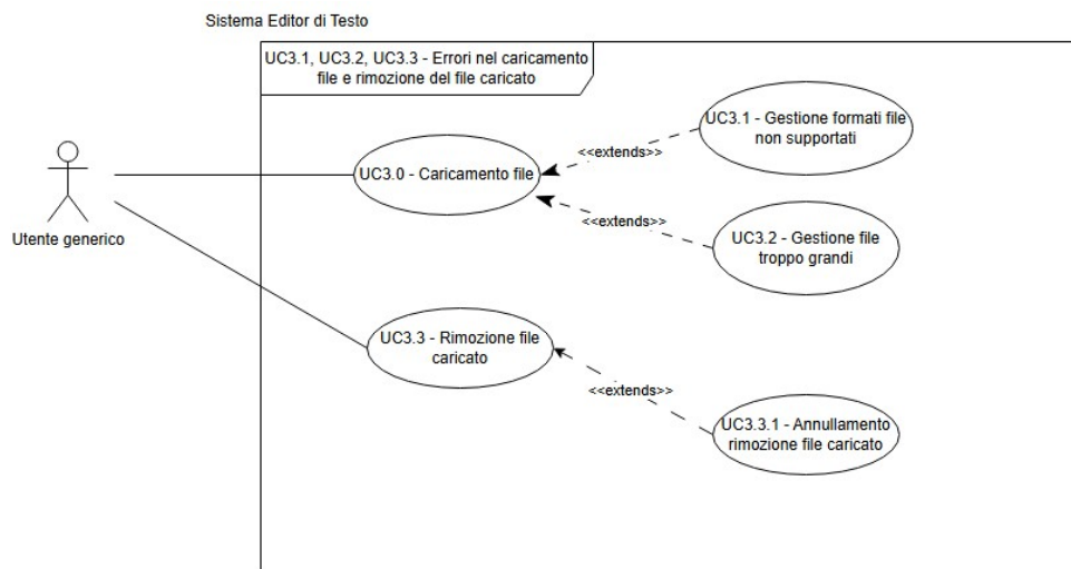
Figura 25: Diagramma dei casi d'uso UC-3.1, 3.2, 3.3
