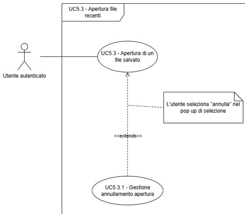
Figura 31: Diagramma dei casi d'uso UC-5.3, 5.3.1
