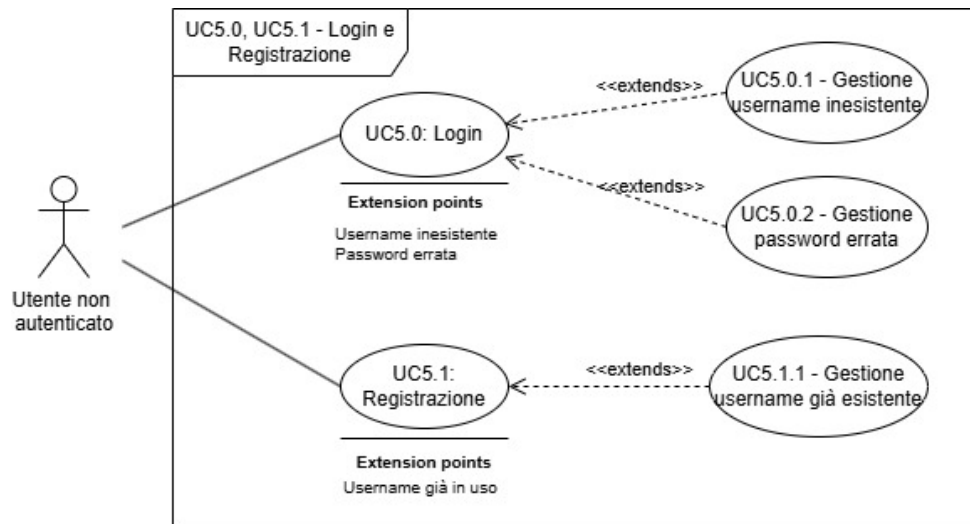
Figura 29: Diagramma dei casi d'uso UC-5.0, 5.0.*, 5.1, 5.1.*
