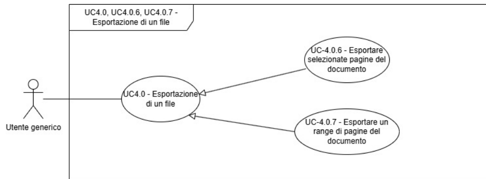
Figura 27: Diagramma dei casi d'uso UC-4.0, UC-4.0.6, UC-4.0.7
