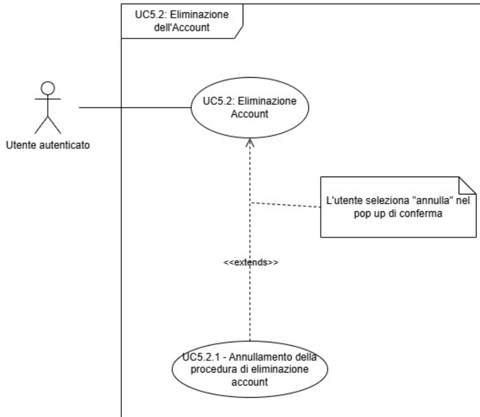
Figura 30: Diagramma dei casi d'uso UC-5.2, 5.2.1
