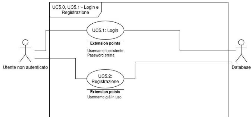
Figura 17: Diagramma dei casi d'uso UC-5.0, UC-5.1
