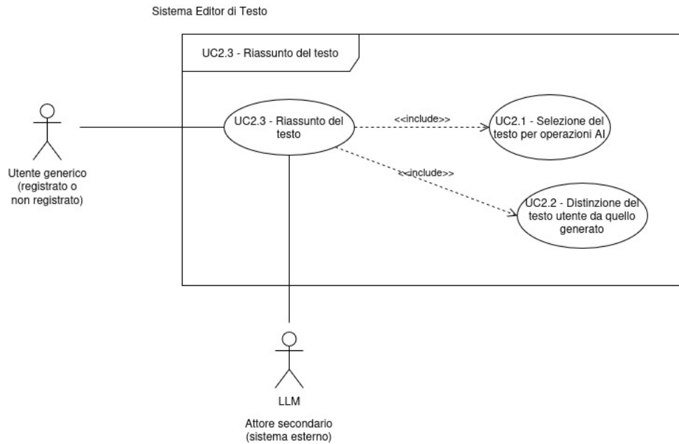
Figura 11: Diagramma del caso d'uso UC-2.3
