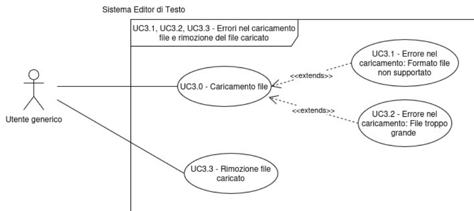
Figura 13: Diagramma dei casi d'uso UC-3.1, 3.2, 3.3
