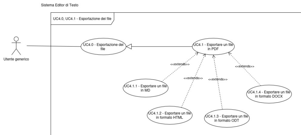
Figura 14: Diagramma dei casi d'uso UC-4.0, UC-4.1, UC-4.1.*
