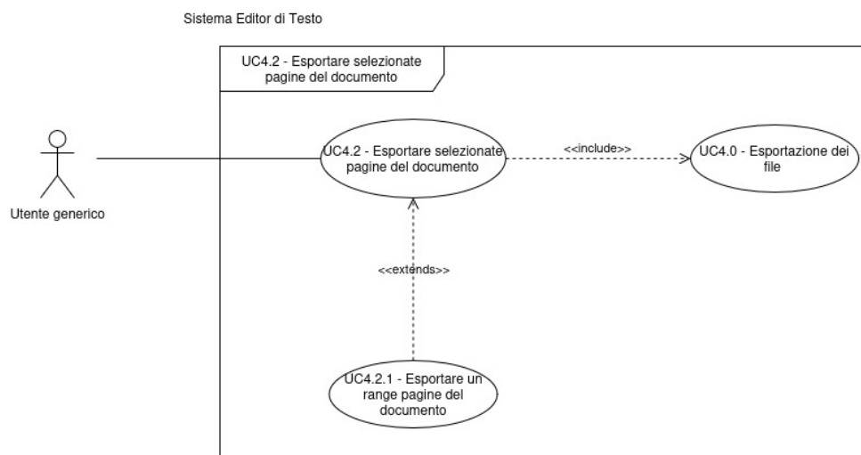
Figura 15: Diagramma dei casi d'uso UC-4.2, UC-4.2.1
