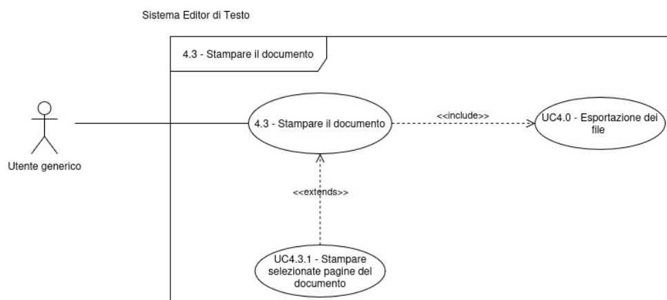
Figura 16: Diagramma dei casi d'uso UC-4.3, UC-4.3.1
