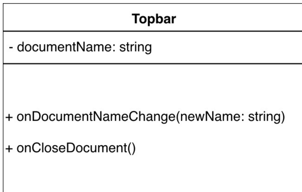
Figura 2: UML TopBar
