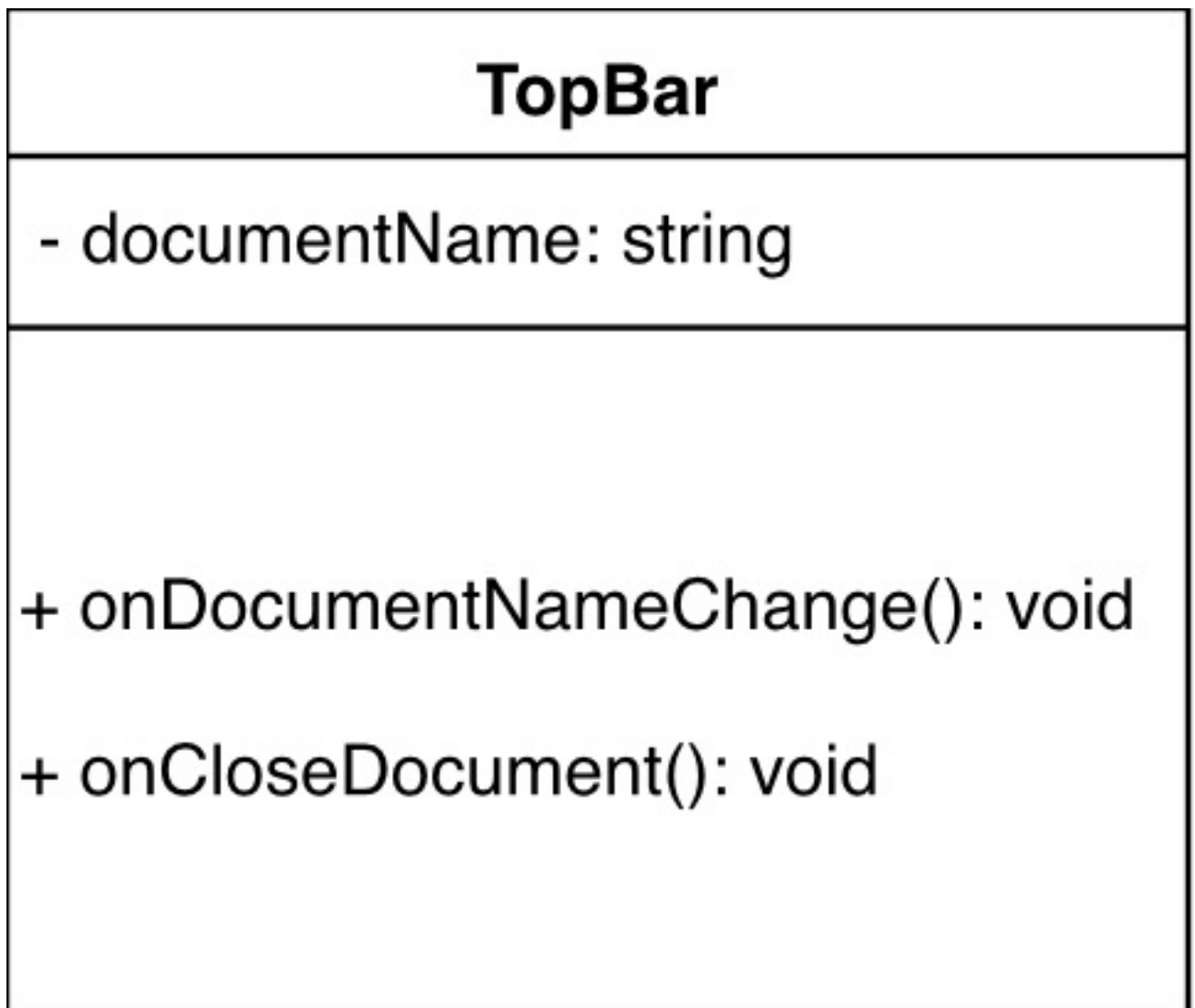
Figura 1: UML TopBar
