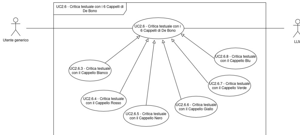
Figura 17: Diagramma dei casi d'uso UC-2.6.3 - 2.6.8
