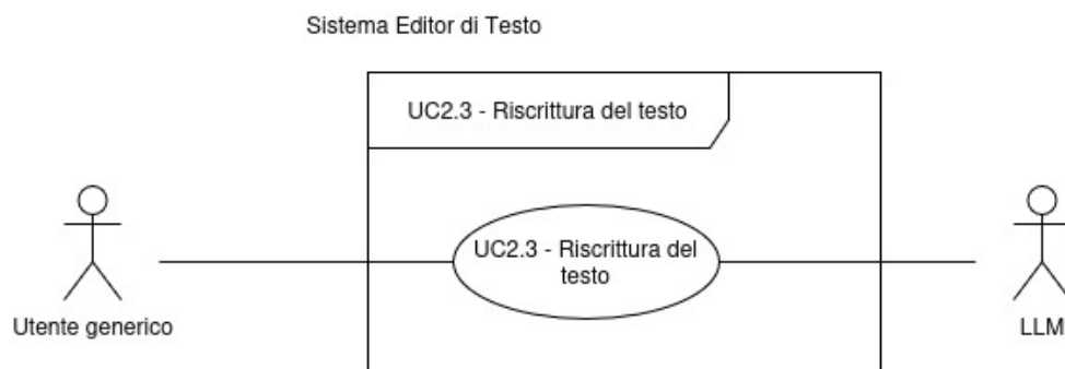
Figura 13: Diagramma dei casi d'uso UC-2.3
