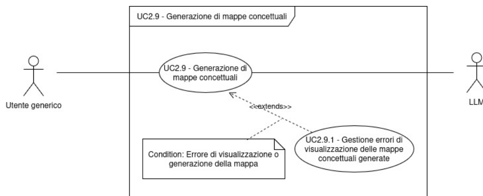
Figura 20: Diagramma dei casi d'uso UC-2.9, 2.9.1
