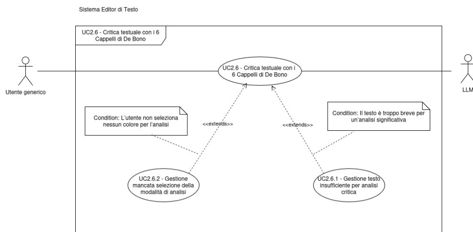
Figura 16: Diagramma dei casi d'uso UC-2.6, 2.6.1, 2.6.2
