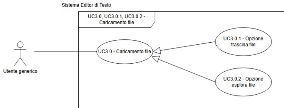
Figura 22: Diagramma dei casi d'uso UC-3.0, 3.0.1, 3.0.2
