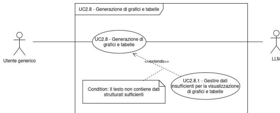
Figura 19: Diagramma dei casi d'uso UC-2.8, 2.8.1
