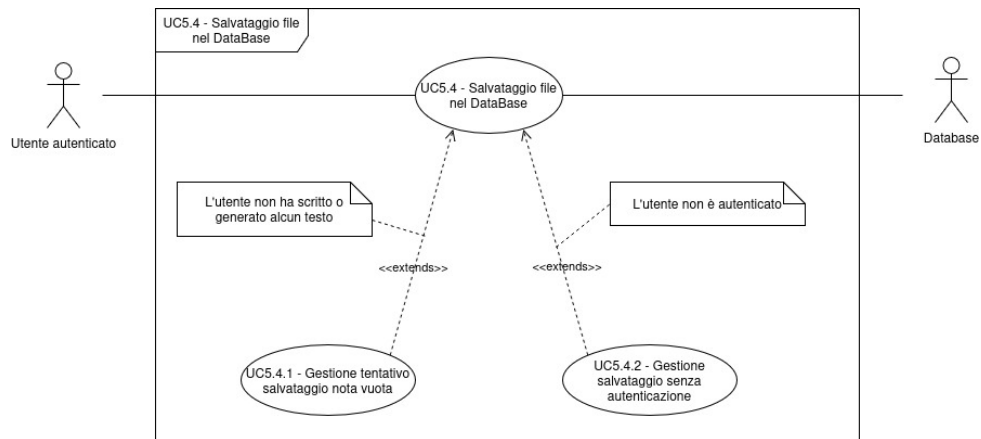
Figura 30: Diagramma dei casi d'uso UC-5.4, 5.4.1, 5.4.2
