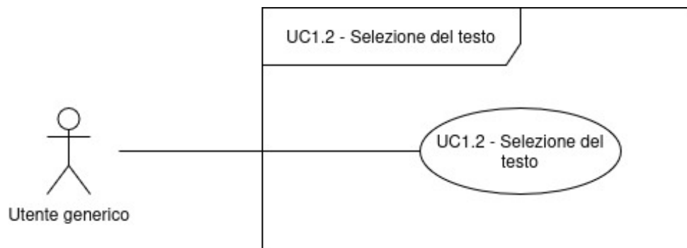
Figura 3: Diagramma dei casi d'uso UC-1.2
