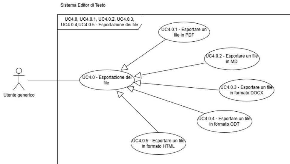
Figura 24: Diagramma dei casi d'uso UC-4.0, UC-4.0.1, UC-4.0.2, UC-4.0.3, UC-4.0.4, UC-4.0.5*
