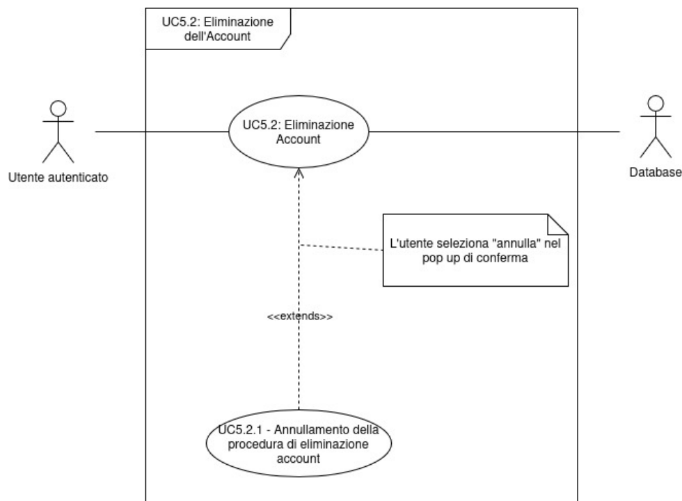
Figura 28: Diagramma dei casi d'uso UC-5.2, 5.2.1
