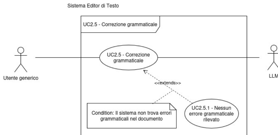
Figura 15: Diagramma dei casi d'uso UC-2.5, 2.5.1
