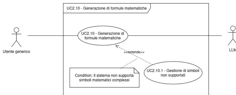
Figura 21: Diagramma dei casi d'uso UC-2.10, 2.10.1
