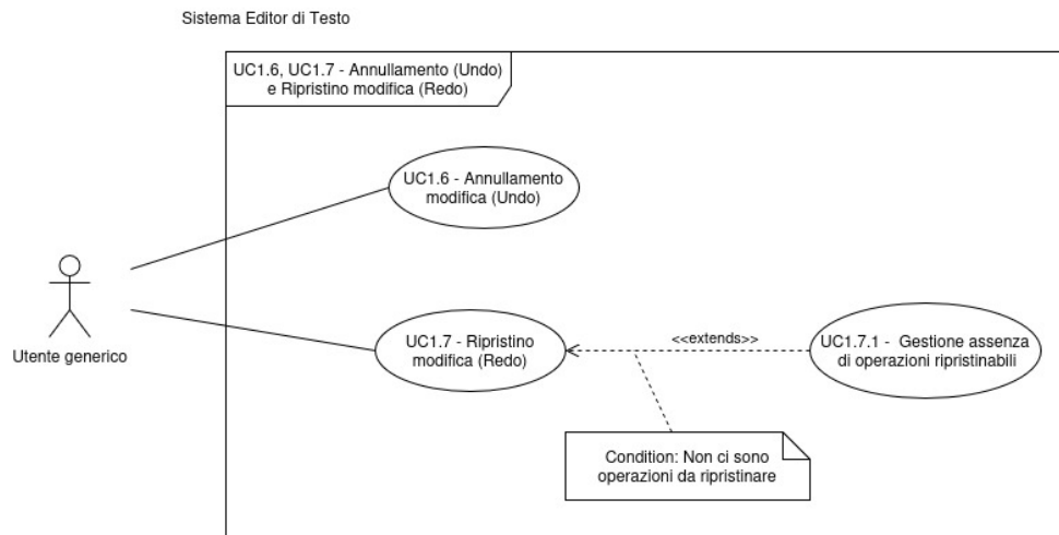
Figura 5: Diagramma dei casi d'uso UC-1.6, 1.7 e estensioni
