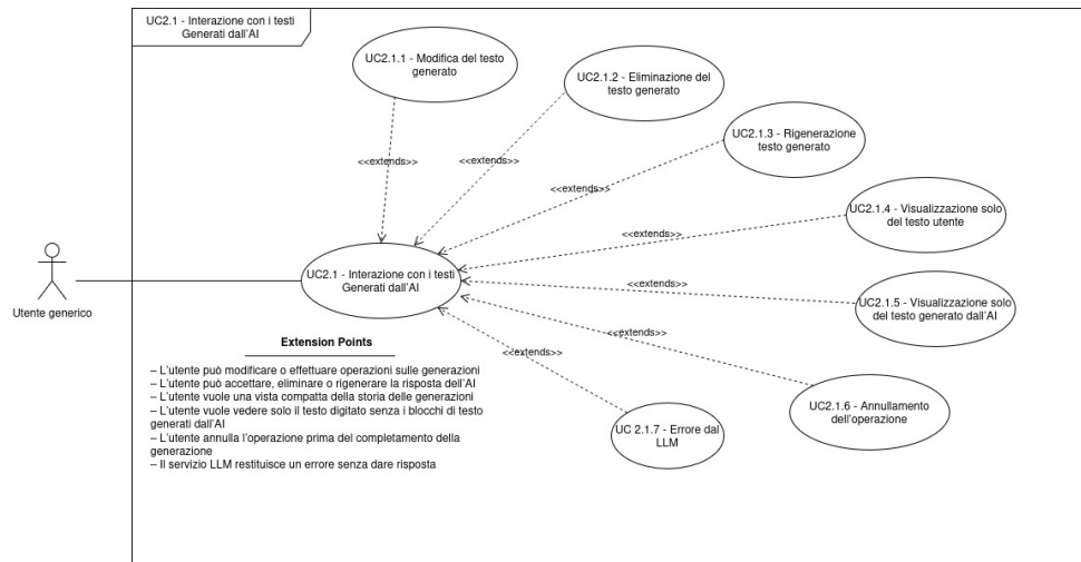
Figura 11: Diagramma dei casi d'uso UC-2.1, 2.1.*
