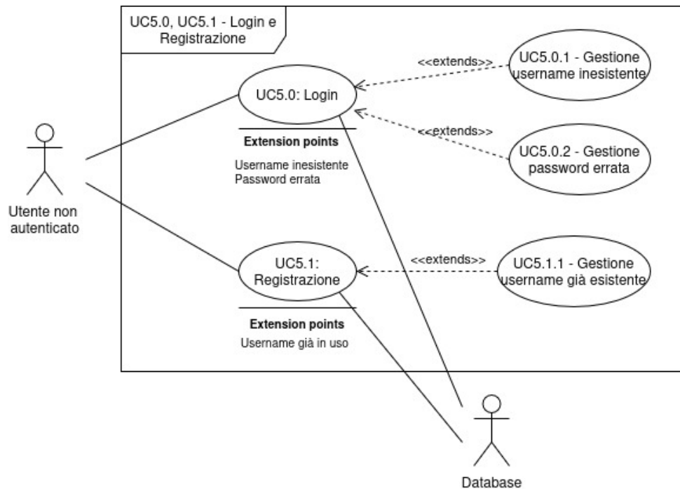
Figura 27: Diagramma dei casi d'uso UC-5.0, 5.0.*, 5.1, 5.1.*
