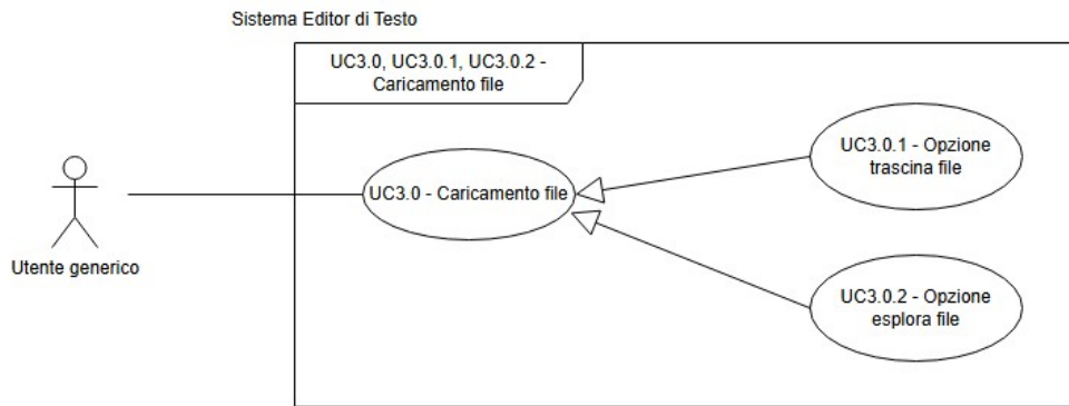
Figura 23: Diagramma dei casi d'uso UC-3.0, 3.0.1, 3.0.2
