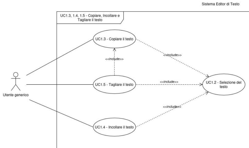
Figura 4: Diagramma dei casi d'uso UC-1.3, 1.4, 1.5
