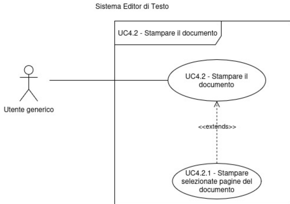
Figura 27: Diagramma dei casi d'uso UC-4.2, UC-4.2.1
