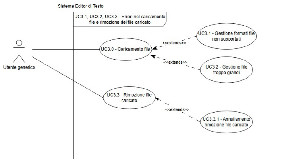
Figura 24: Diagramma dei casi d'uso UC-3.1, 3.2, 3.3
