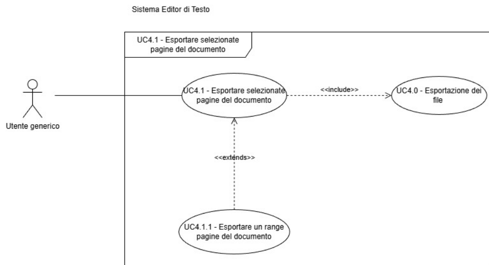
Figura 26: Diagramma dei casi d'uso UC-4.1, UC-4.1.1
