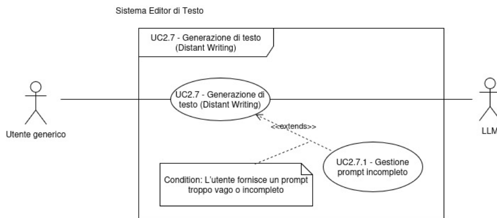
Figura 19: Diagramma dei casi d'uso UC-2.7, 2.7.1
