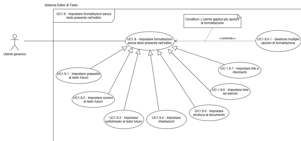
Figura 8: Diagramma dei casi d'uso UC-1.9.*
