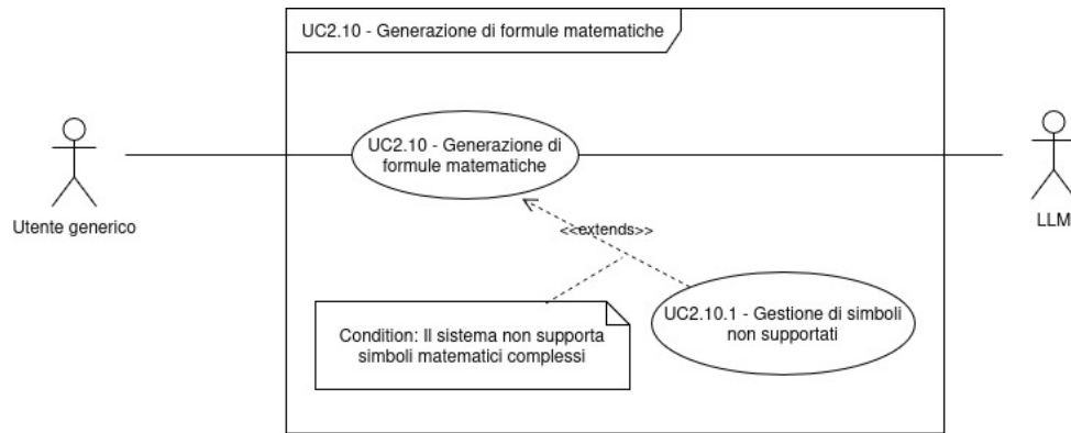
Figura 22: Diagramma dei casi d'uso UC-2.10, 2.10.1
