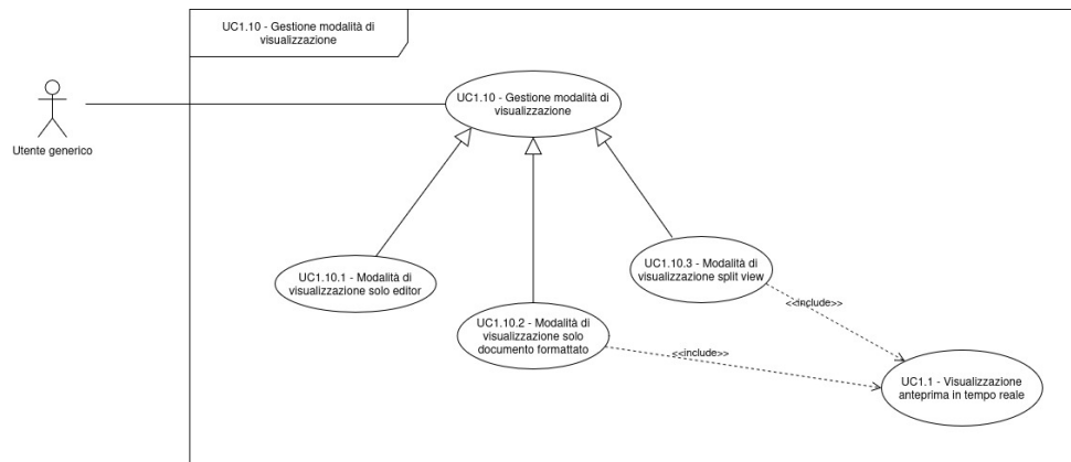
Figura 9: Diagramma dei casi d'uso UC-1.10, 1.10.*
