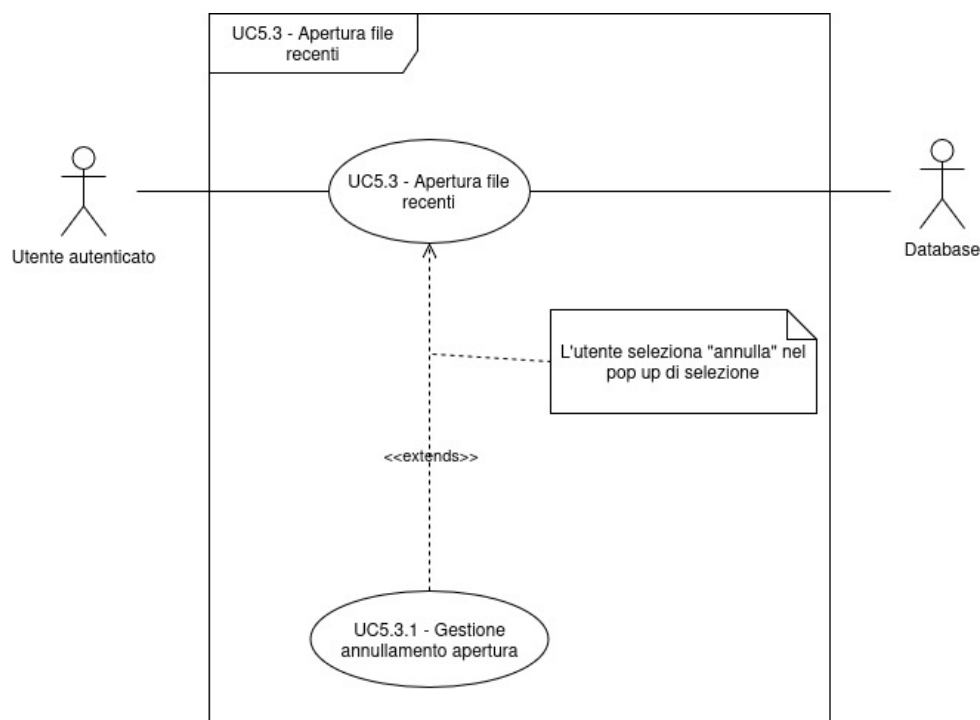
Figura 30: Diagramma dei casi d'uso UC-5.3, 5.3.1
