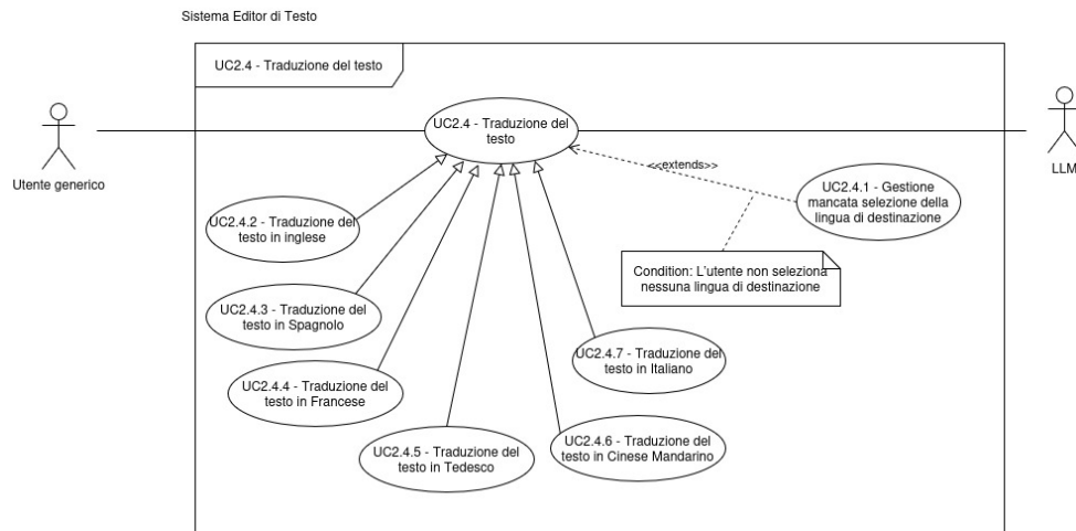
Figura 15: Diagramma dei casi d'uso UC-2.4.*
