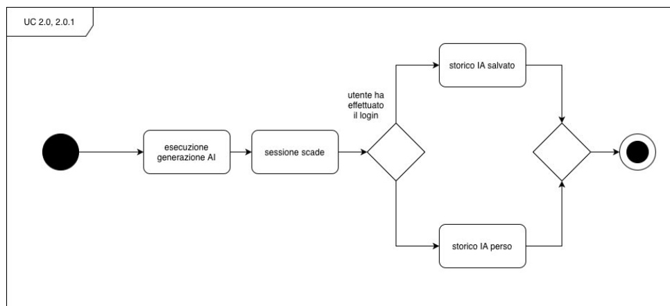
Figura 11: Diagramma delle attività UC-2.0, 2.0.1
