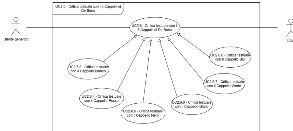
Figura 18: Diagramma dei casi d'uso UC-2.6.3 - 2.6.8
