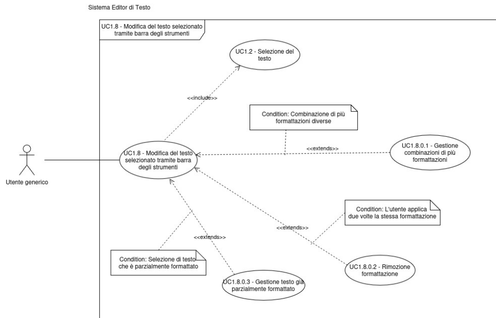
Figura 6: Diagramma dei casi d'uso UC-1.8.0, 1.8.0.1, 1.8.0.2, 1.8.0.3
