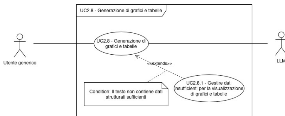
Figura 20: Diagramma dei casi d'uso UC-2.8, 2.8.1
