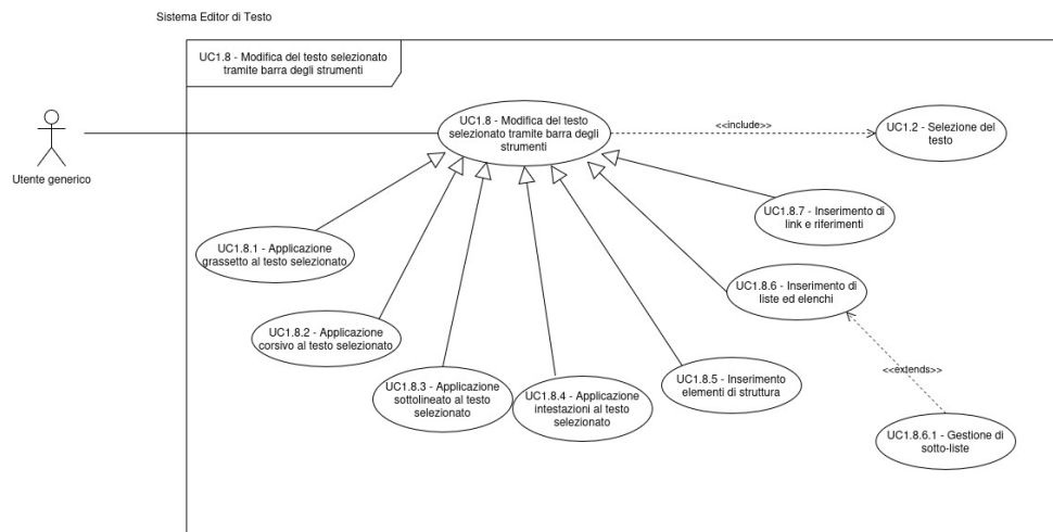
Figura 7: Diagramma dei casi d'uso UC-1.8.*
