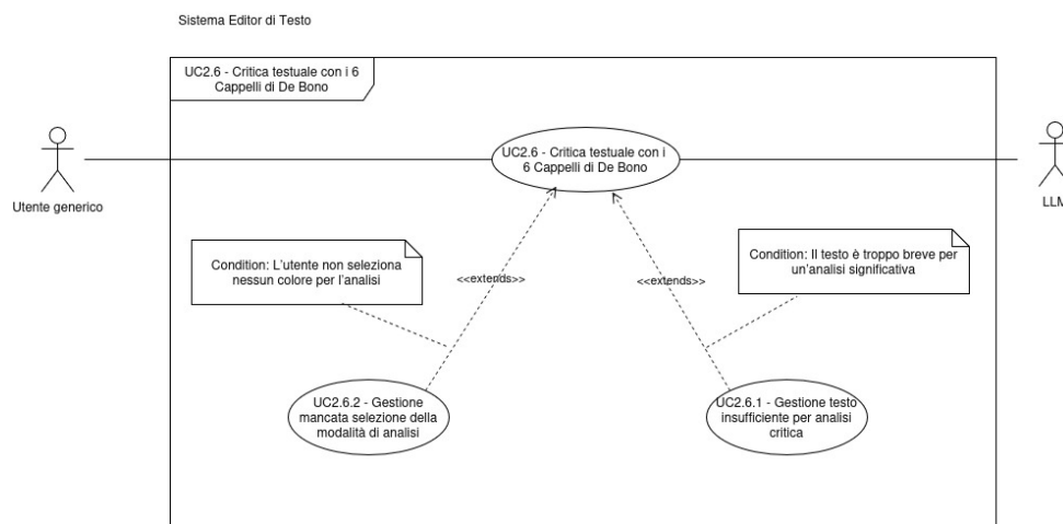
Figura 17: Diagramma dei casi d'uso UC-2.6, 2.6.1, 2.6.2
