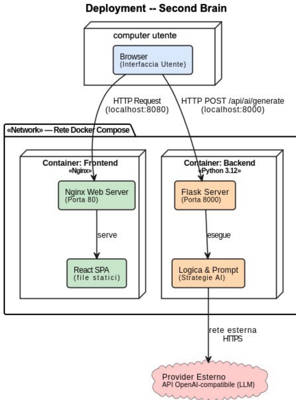
Figura 1: Rappresentazione dell'architettura di deployment tramite Docker Compose G
