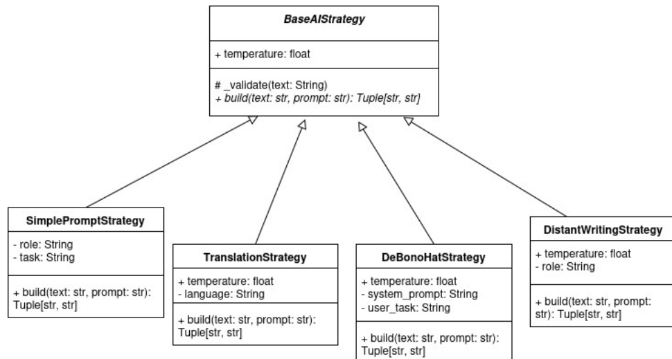
Figura 4: Diagramma UML: Strategy pattern applicato alle operazioni AI
