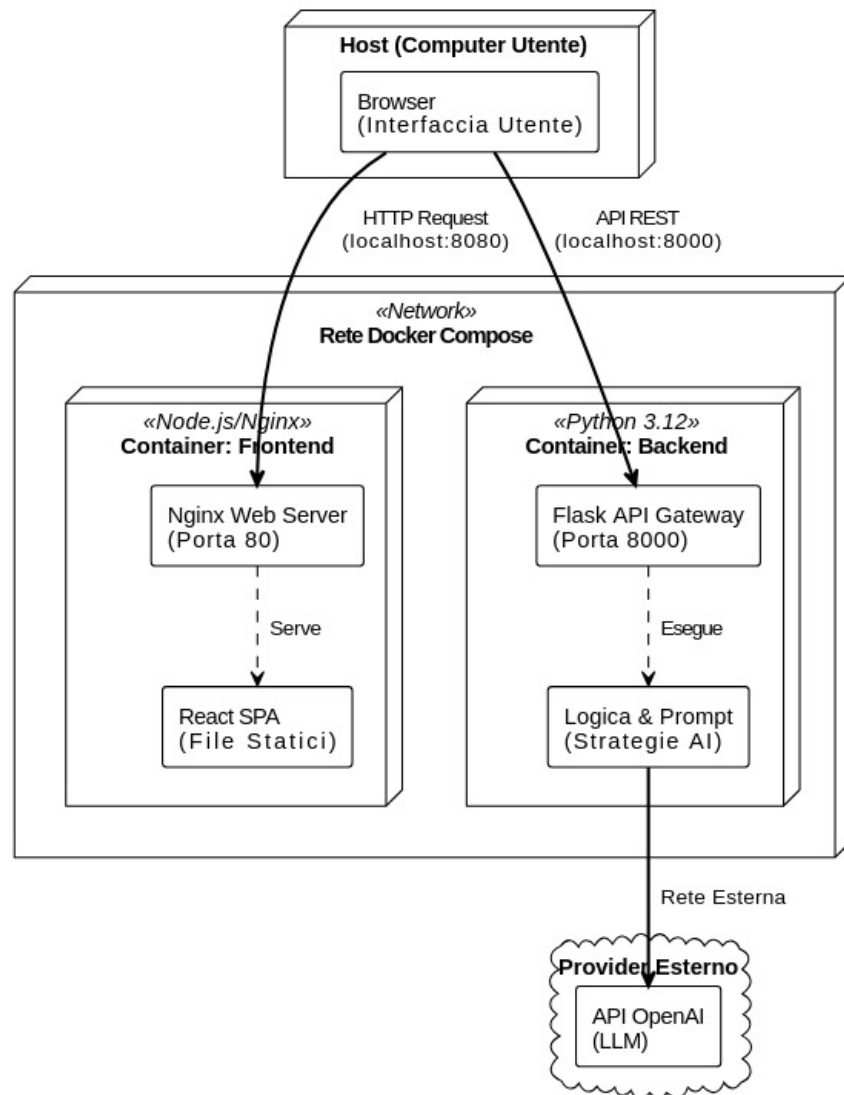
Figura 1: Rappresentazione dell'architettura di deployment tramite Docker Compose
