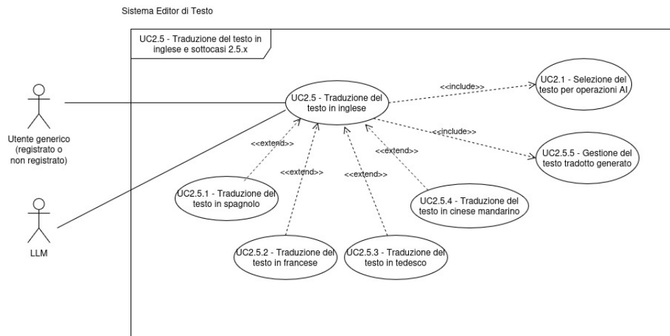
Figura 5: Diagramma dei casi d'uso UC-2.5.*
