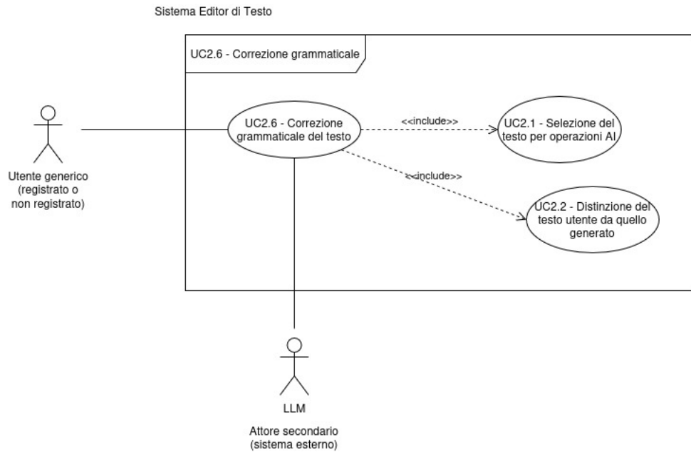
Figura 6: Diagramma del caso d'uso UC-2.6
