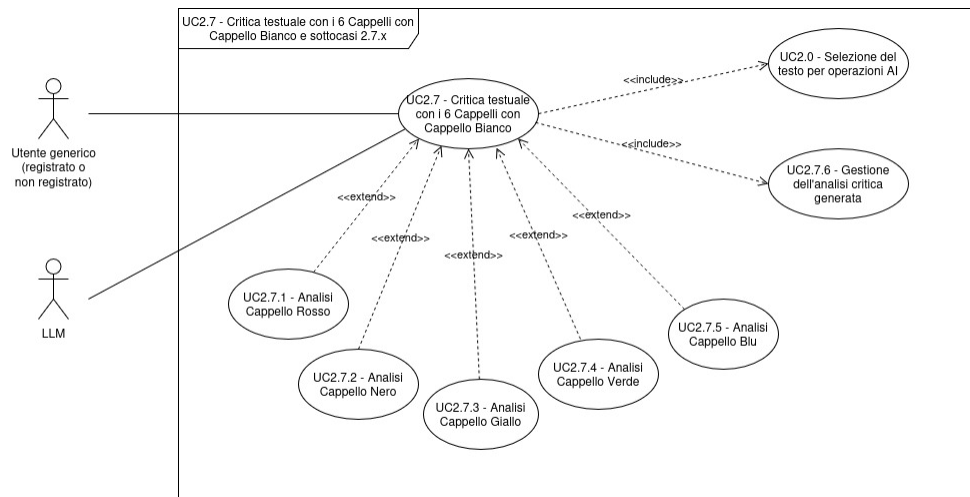
Figura 7: Diagramma dei casi d'uso UC-2.7.*
