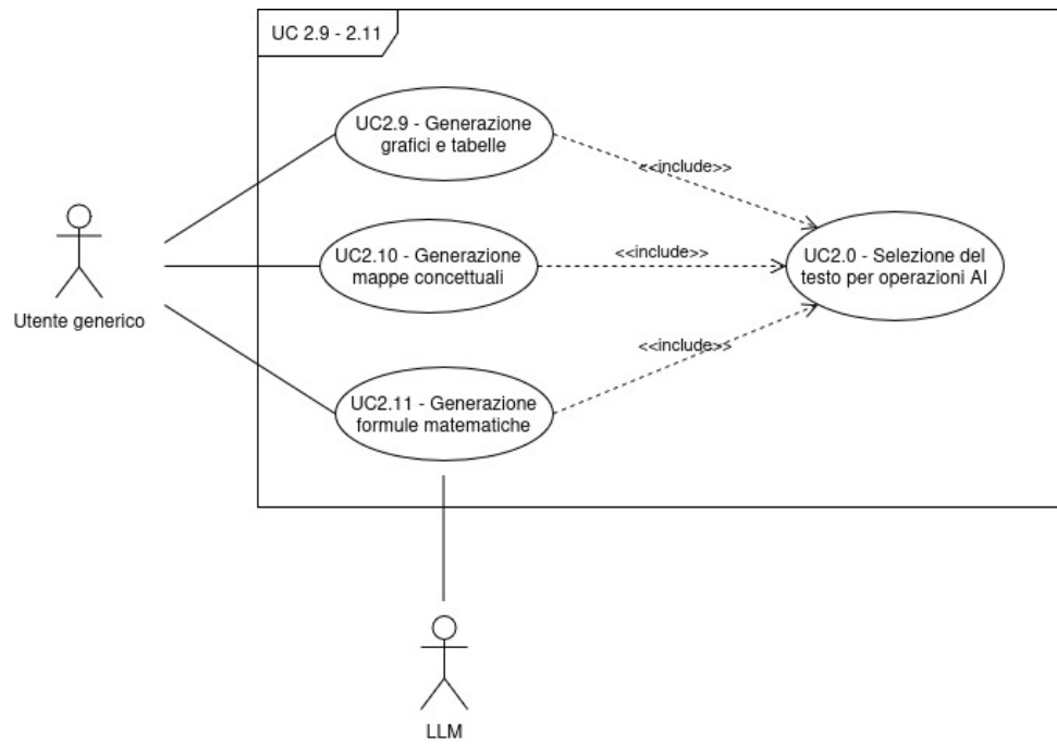
Figura 9: Diagramma dei casi d'uso UC-2.9, UC-2.10, UC2.11 (opzionali)
