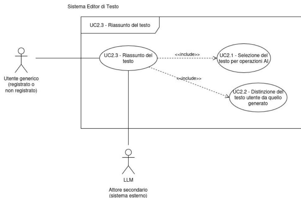
Figura 3: Diagramma del caso d'uso UC-2.3
