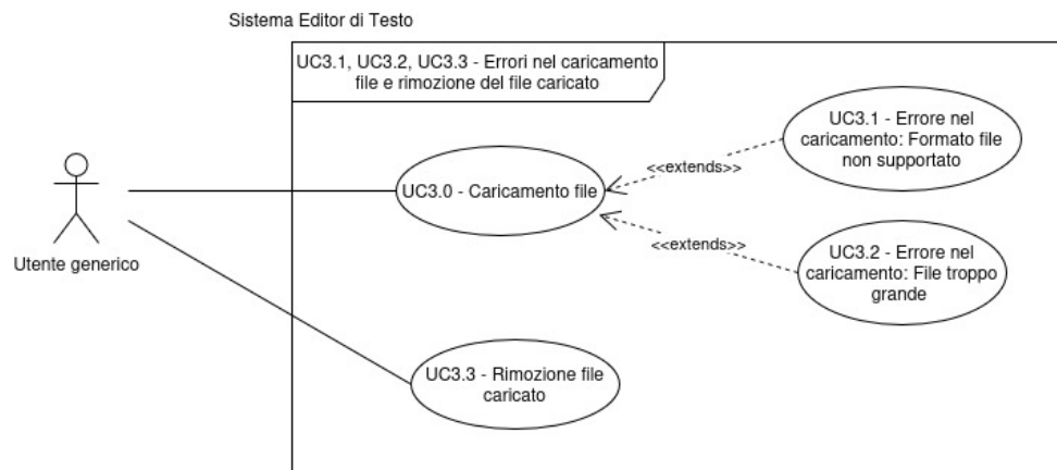
Figura 11: Diagramma dei casi d'uso UC-3.1, 3.2, 3.3
