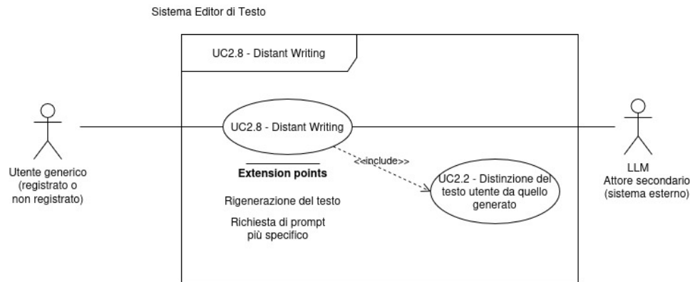
Figura 8: Diagramma del caso d'uso UC-2.8
