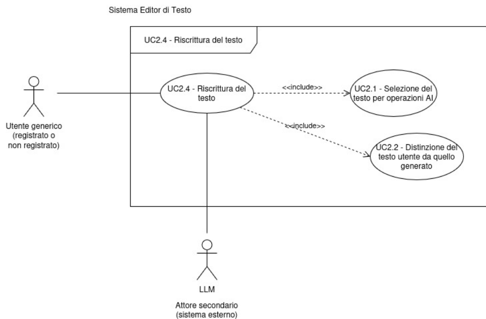
Figura 4: Diagramma del caso d'uso UC-2.4
