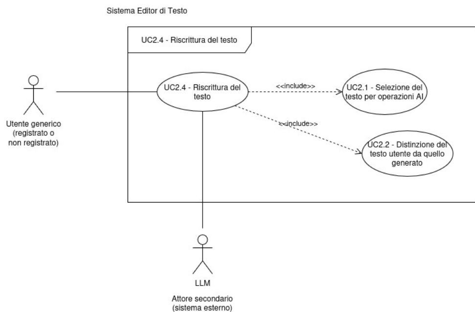
Figura 8: Diagramma del caso d'uso UC-2.4
