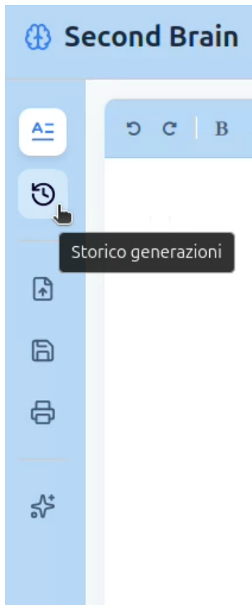
Figura 4: Navigazione
