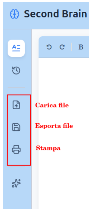
Figura 5: Gestione file
