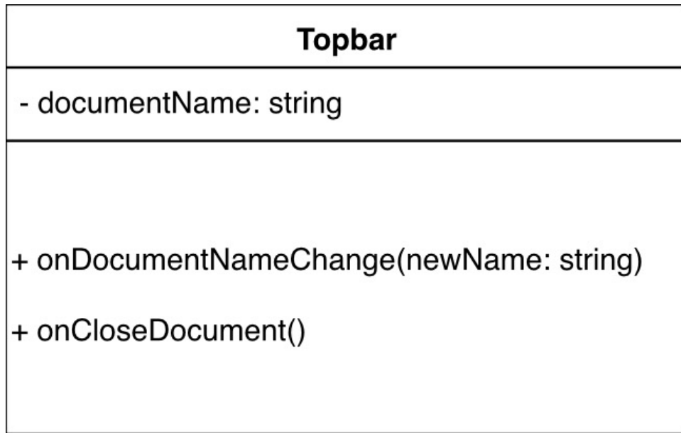
Figura 5: UML TopBar
