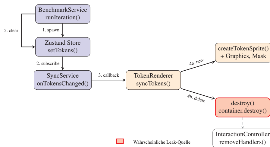
Abbildung 4.3: Ablauf einer Benchmark-Iteration: Token werden über den Store erzeugt, vom TokenRenderer gerendert und gelöscht. Die rot markierte destroy() -Phase ist die wahrscheinliche Quelle des Memory-Leaks.
