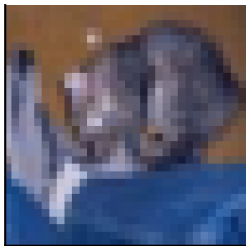
Grad-CAM, clean
