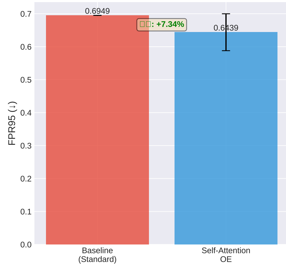
FPR95 (↓) Comparison
