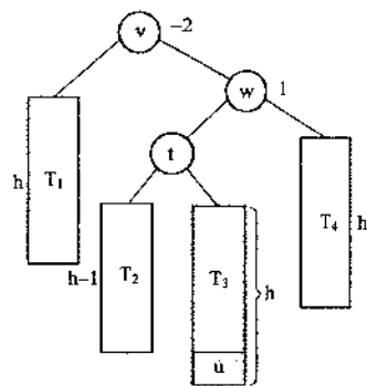
图 8-19 插入结点后失衡的树一
