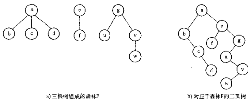
图 5-32 森林与二叉树的转换示例
