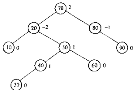
图 8-28 插入 30 后失平衡的树
