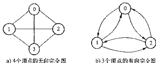
图 6-2 完全图示例
