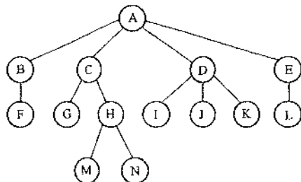
图 5-33 树 T
