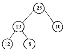
图 7-14 最大堆
