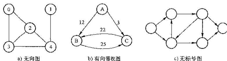
图 6-1 图的示例
