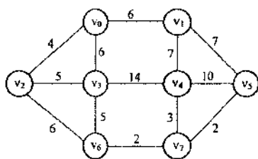
图 6-28 带权图 G
