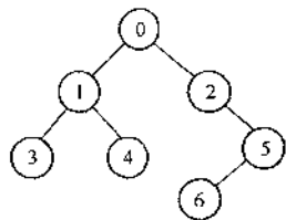
图 5-10 二叉树 T
