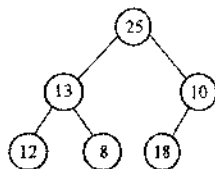
图 7-15 放置新元素 18
