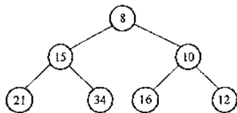
图 7-13 初始最小堆
