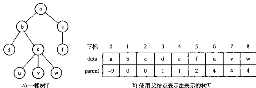
图 5-26 树 T 及其父结点表示
