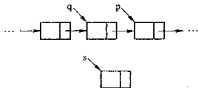
图 2-10 单链表 L 中部分结点及待插入结点的初始状态
