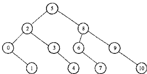
图 8-5 折半查找判定树
