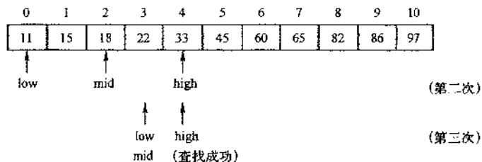
图 8-3 在前半区间查找 22 的过程
