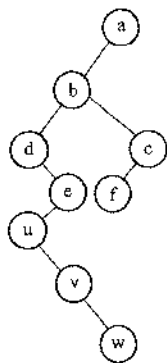
图 5-31 对应于图 5-26a 所示树 T 的二叉树
