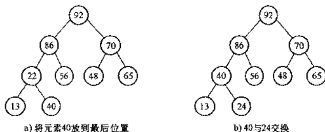
图 5-23 在最大堆中插入新元素
