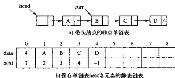
图 2-17 单链表 head 及静态链表
