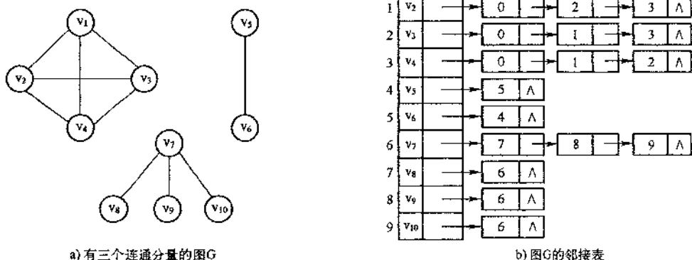
图 6-12 求无向图 G 的连通分量示例
