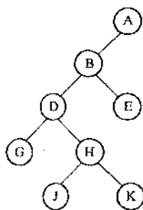
图 5-14 二叉树 T
