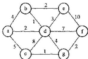
图 6-26 无向带权图
