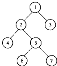
图5-17 二叉树 T
