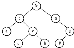
图 5-43 解答题 6 的图
