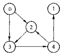
图 6-4 路径示例
