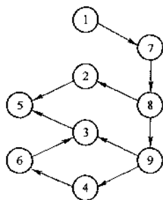
图 6-22 AOV 网
