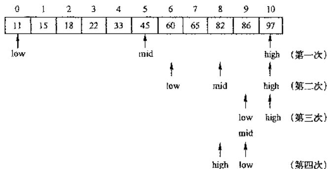
图 8-4 查找 85 的过程
