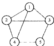
图 6-29 无向图
