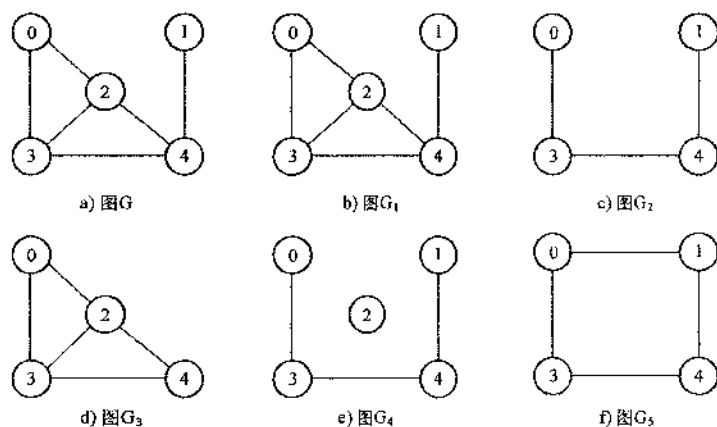
图 6-3 子图示例
