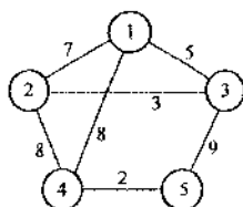
图 6-30 带权无向图
