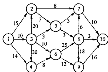
图 6-33 AOE 网
