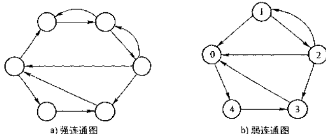
图 6-5 有向连通图
