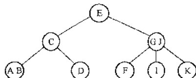
图 8-30 3 阶 B 树
