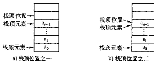
图 3-4 栈顶位置 top 的两种定义方式
