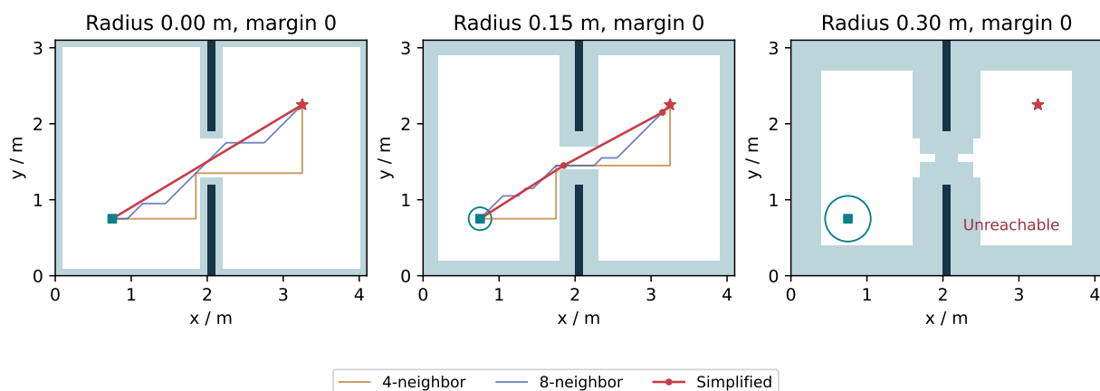
图 11.1: 深色是给定的隔墙, 浅蓝是额外阻塞的配置空间格子, 白色可规划。绿方块为起点, 红星为目标; 绿圆保持真实半径与坐标等比例。红线为八邻接结果的简化。
