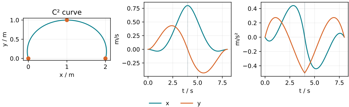
图 14.2: 两个 4 s 分段，连接点 (1,1) m，连接速度 (0.8,0) m/s、加速度 (0,-0.5) m/s 2 。虚线是连接时刻；图形坐标等比例，速度与加速度连续。
