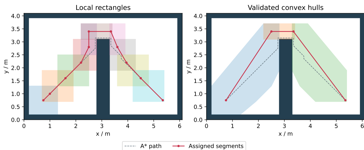
图 13.1: 深色为已膨胀阻塞格, 浅色为走廊, 虚线为原始 A* 路径。红色线段的两端点均分配到同一个凸区域中。两图采用相同坐标比例。
