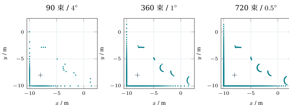
图 5.3: 同一 \text{seed}=42 世界、同一圆心 (-8, -8) 、 \text{yaw}=0 、关闭噪声的有限回波。十字为雷达。点列之间的空白包含光束间隙和被遮挡区域。
