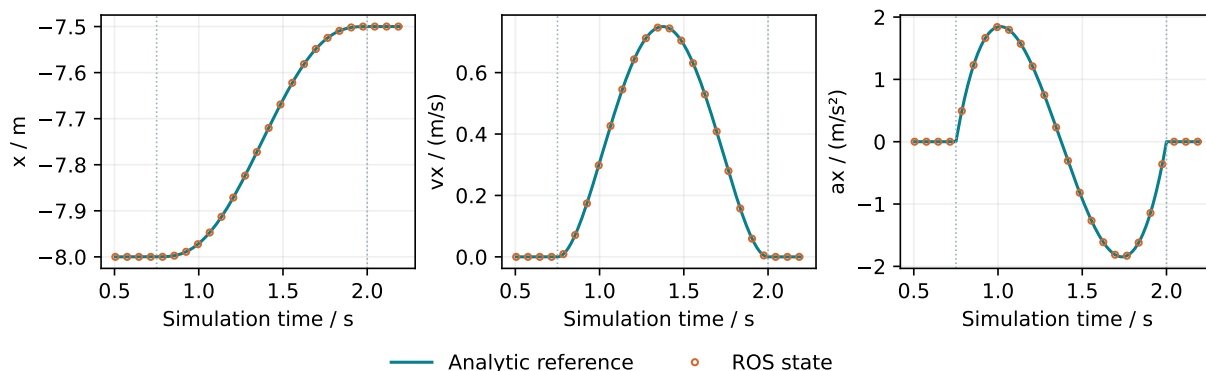
图 14.3: 实际观测地图上执行半圆路线。0.75 s 开始、2 s 结束；实测 p/v/a 与解析参考重合，用空心点区别采样结果与参考曲线。
