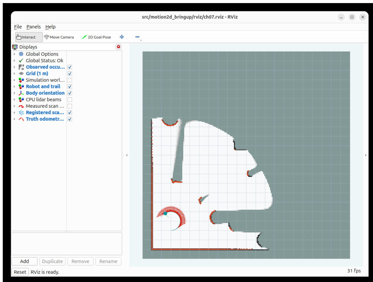
图 7.1: RViz2 中的观测地图。浅色是已观测自由域，深色轮廓是占据证据，灰色是未知。橙色点为当前回波，箭头表示真值里程计位姿。
