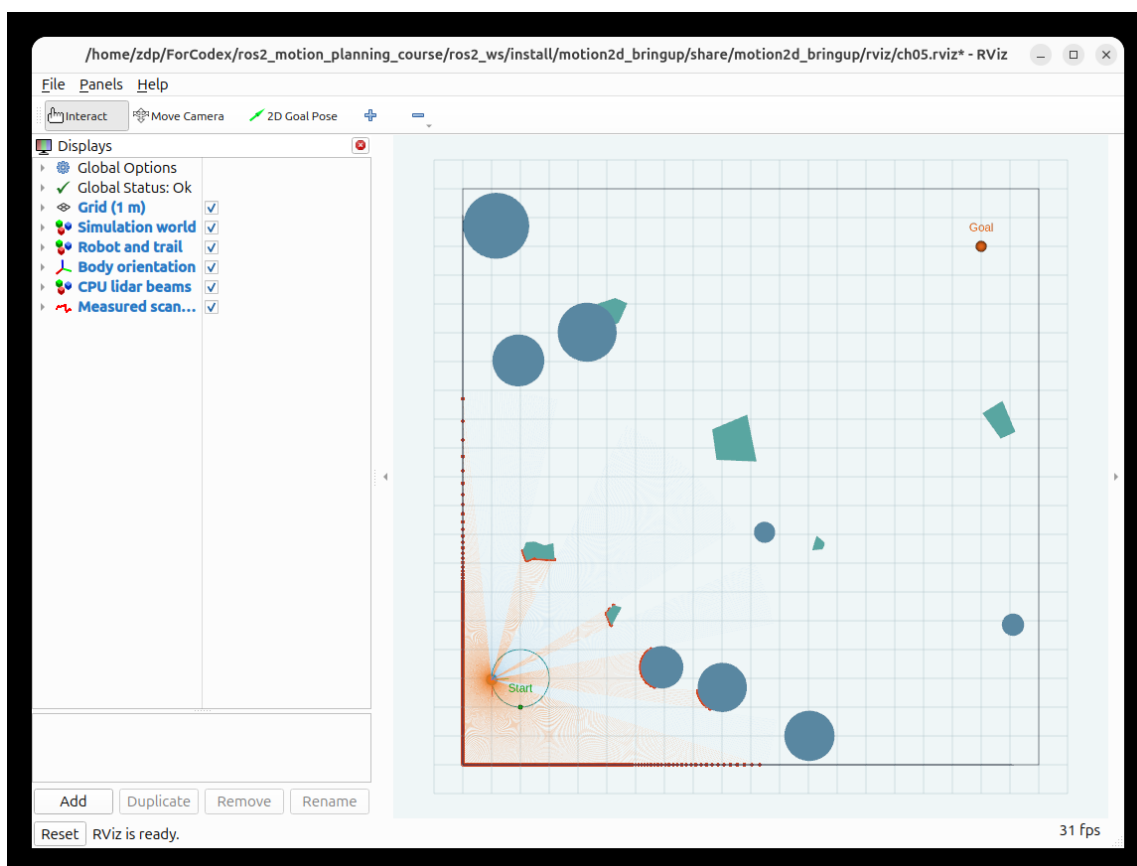
图 5.1: 关闭测距噪声的主机基准画面。橙色线是有效测距射线，红点是 LaserScan 命中点；淡蓝线只表示量程内无回波，障碍后的空间仍可见。
