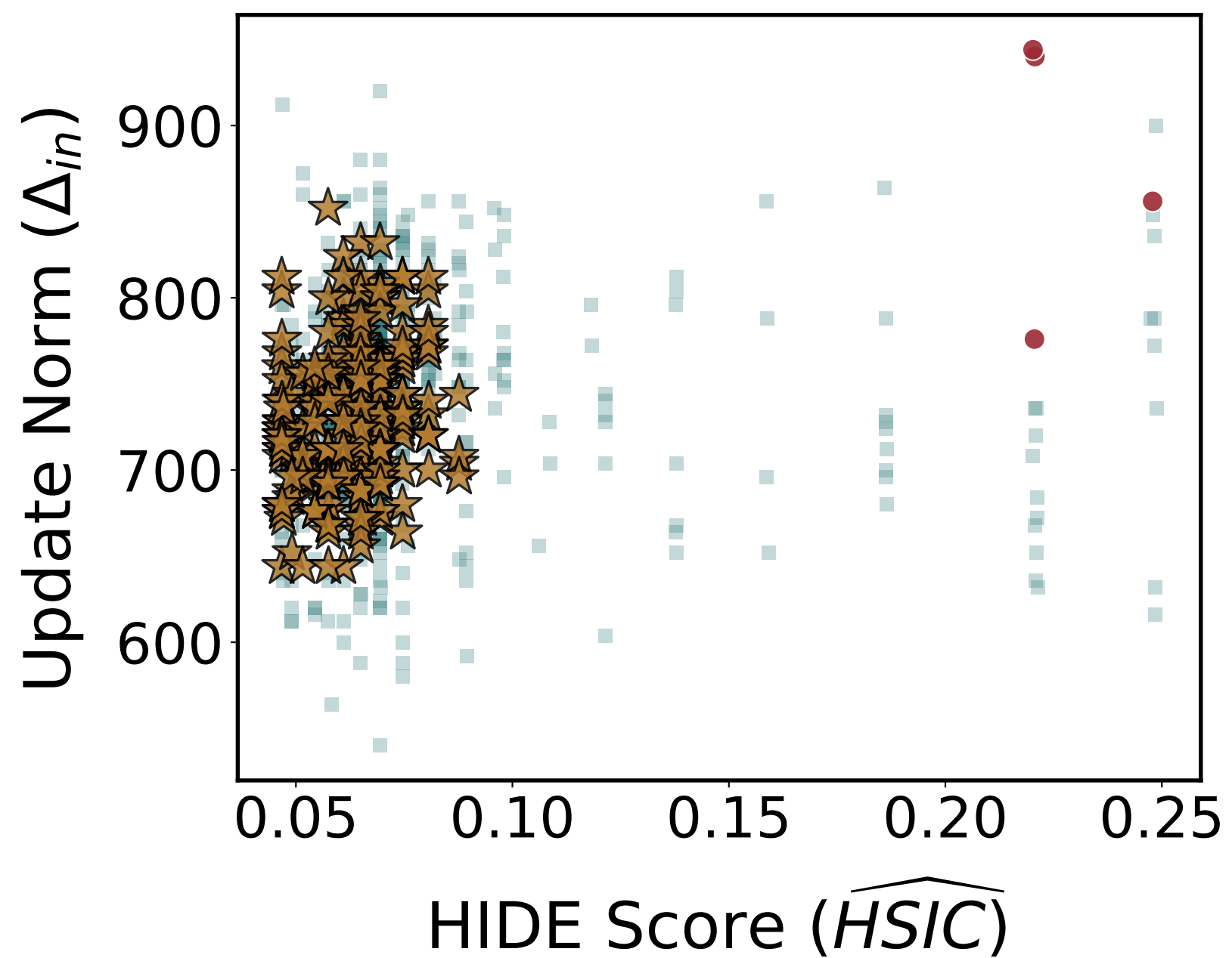
(d) NQ, PCC: 0.091
