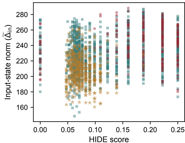
(d) NQ; PCC = 0.367
