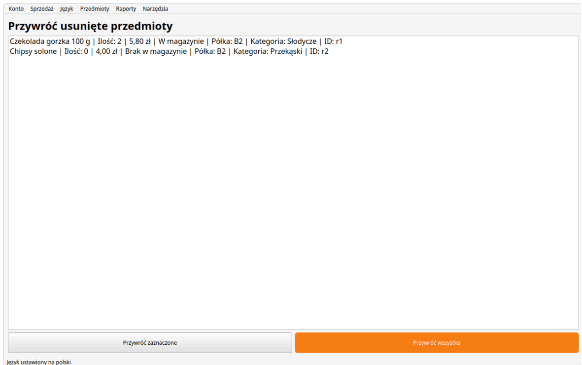
Rysunek 5-3: Cofnij usunięte przedmioty — przywracanie „miękkich” usunięć.
