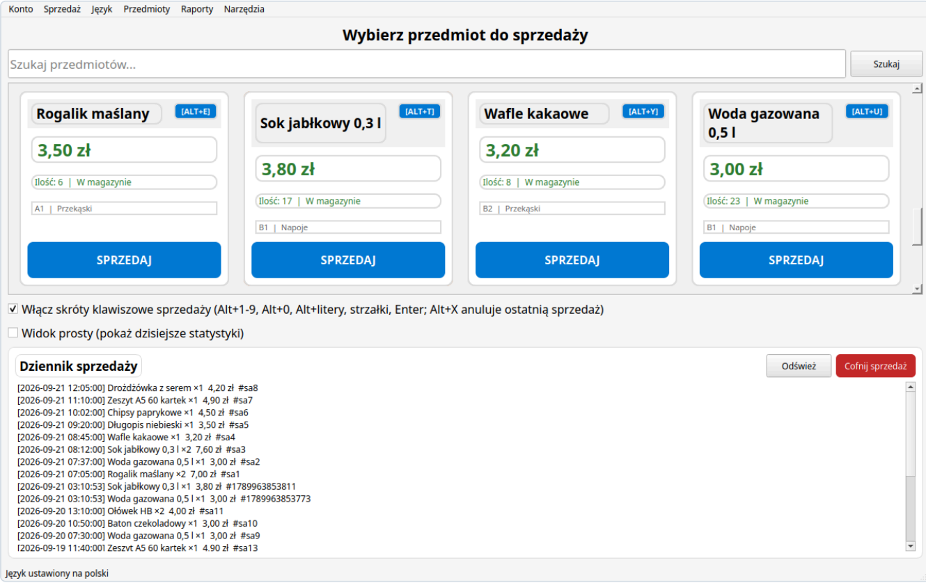
Rysunek 2-1: Strona Sprzedaż — kasa, na której pracujesz cały dzień.
