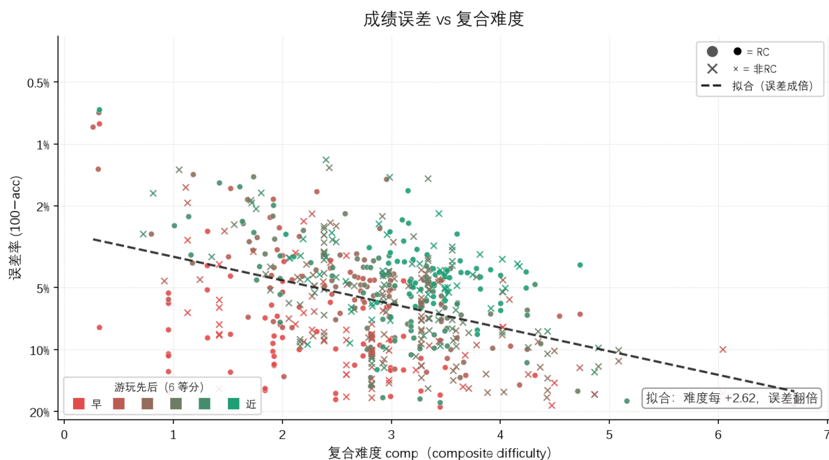
Figure 3: 成绩误差 vs 复合难度。横轴为复合难度 comp; y 轴为误差率 (100 - acc) 对数轴并反转, 越靠上越准。颜色按游玩先后均分为 6 段 (非真实日期线性, 因记录集中在近期); 标记: ● = RC, × = 非 RC; 虚线 = 误差随难度的成倍增长拟合。
