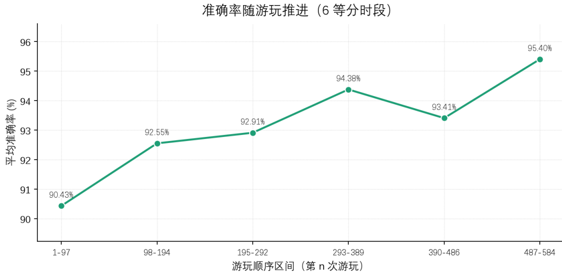
Figure 4: 准确率随游玩推进 (6 等分时段)。横轴为按游玩顺序均分的 6 个等数量区间，纵轴为该区间平均准确率。
