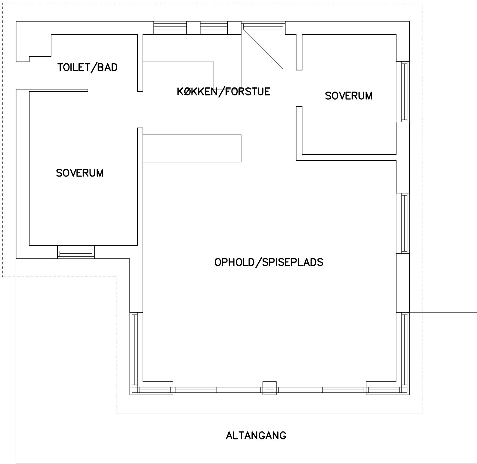
OPMPLINGSPLAN AF STUEETAGEN MÅL 1:50
