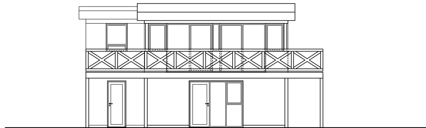
OPMÅLINGSFACADE MOD VEST MÅL 1:100
