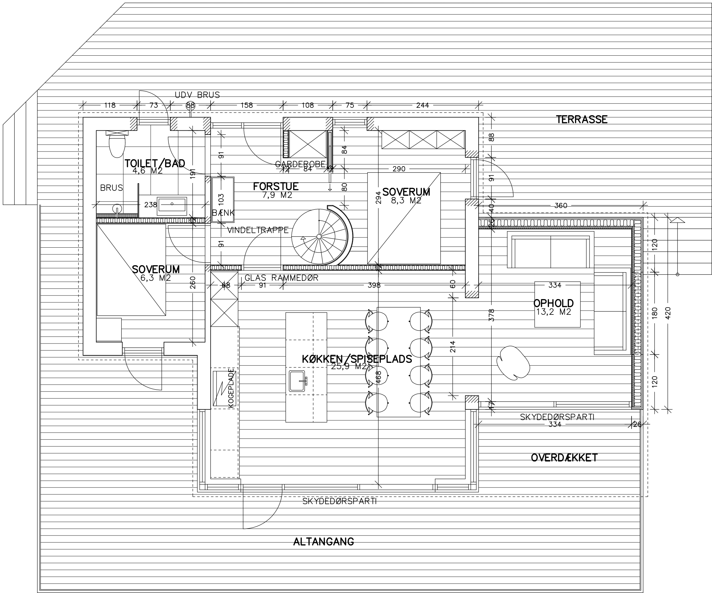
STUEPLAN MÅL 1: 500
