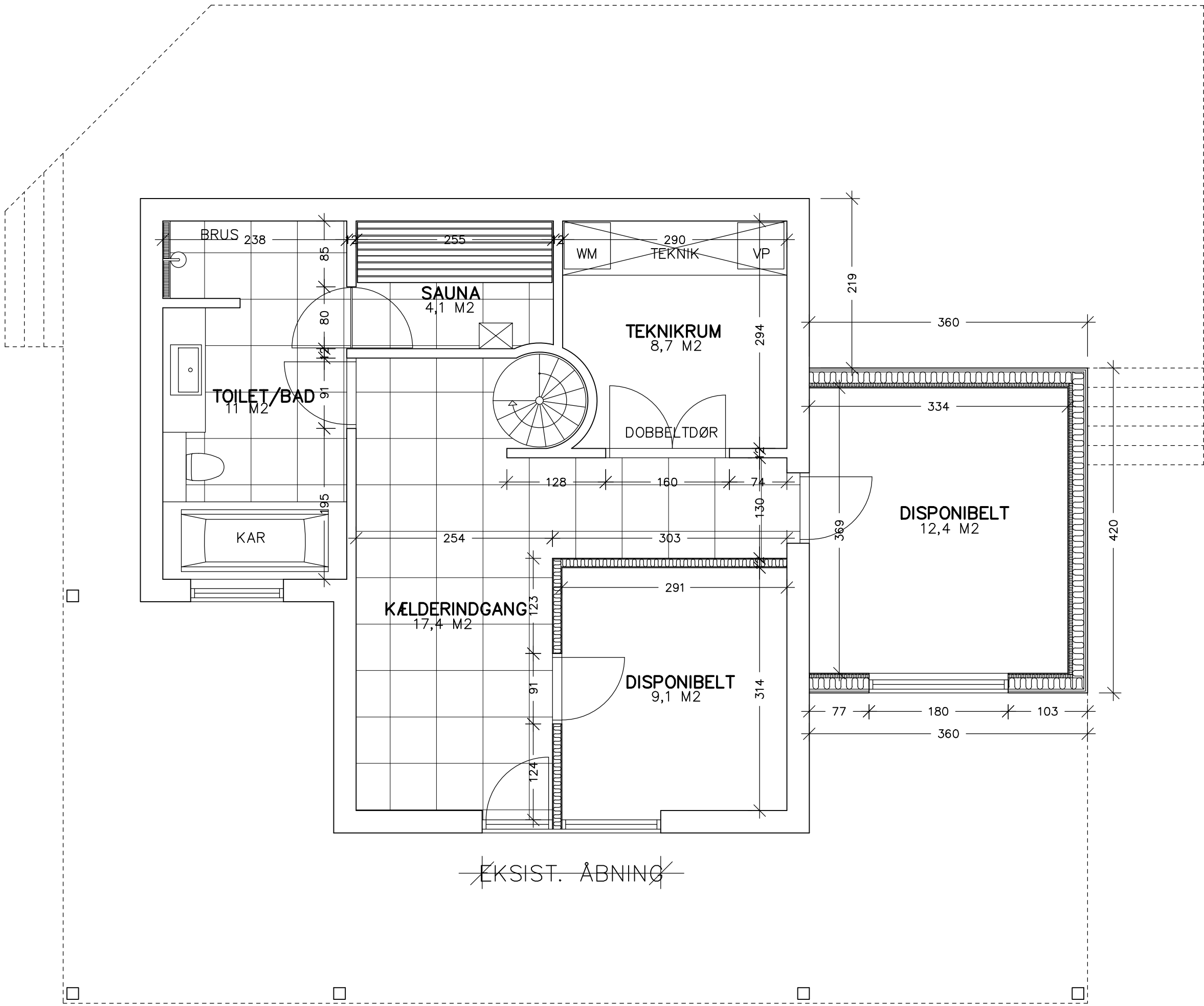
KÆLDERPLAN MÅL 1: 500
