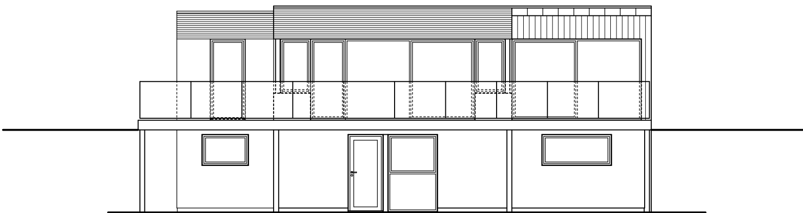
FACADE MOD VEST MÅL 1:100
