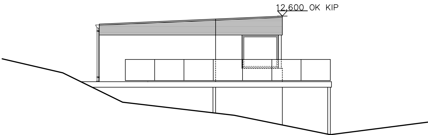
GAVL MOD NORD MÅL 1:100
