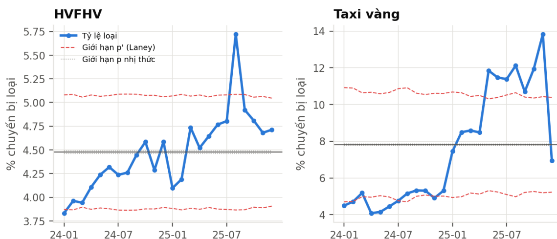
Hình 6.2. Biểu đồ kiểm soát tỷ lệ bản ghi bị loại theo tháng: giới hạn p nhị thức và giới hạn p' của Laney
