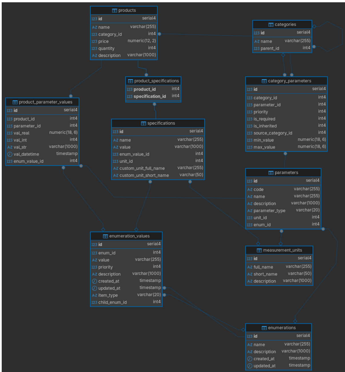
Рисунок 3 — диаграмма классов
