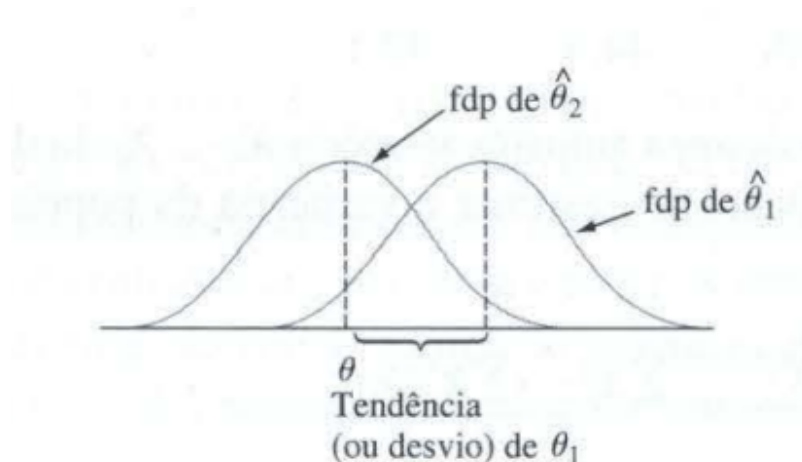
Figura 1. As fdps de um estimador tendencioso \Theta_1 , e um estimador não-tendencioso \Theta_2 , para o parâmetro \Theta .
