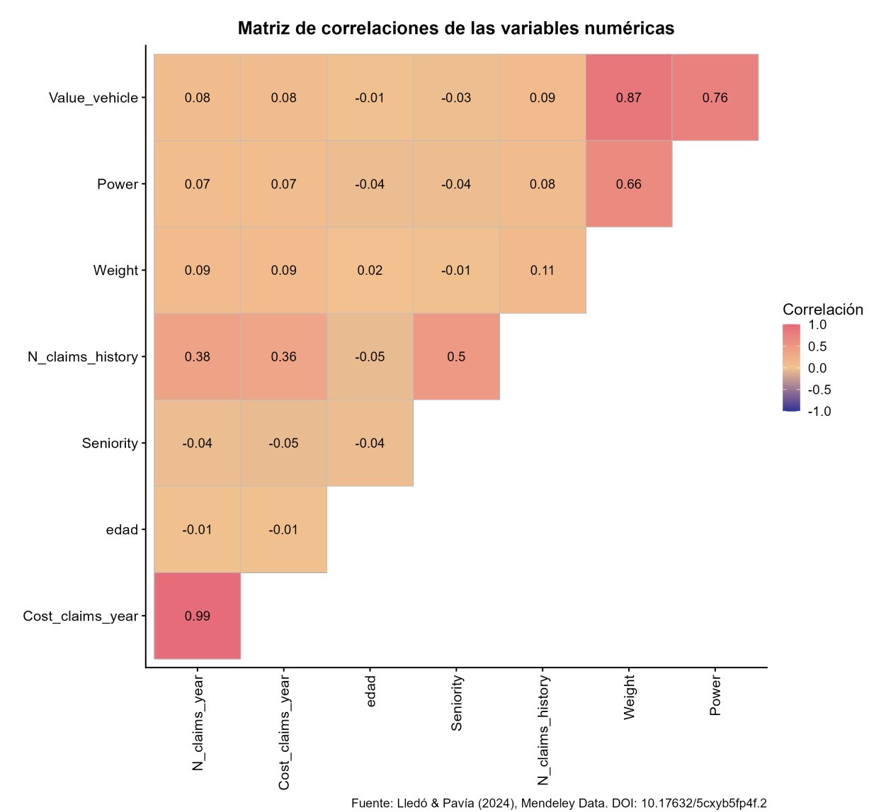
Figura 9: Matriz de correlaciones de las variables numéricas
