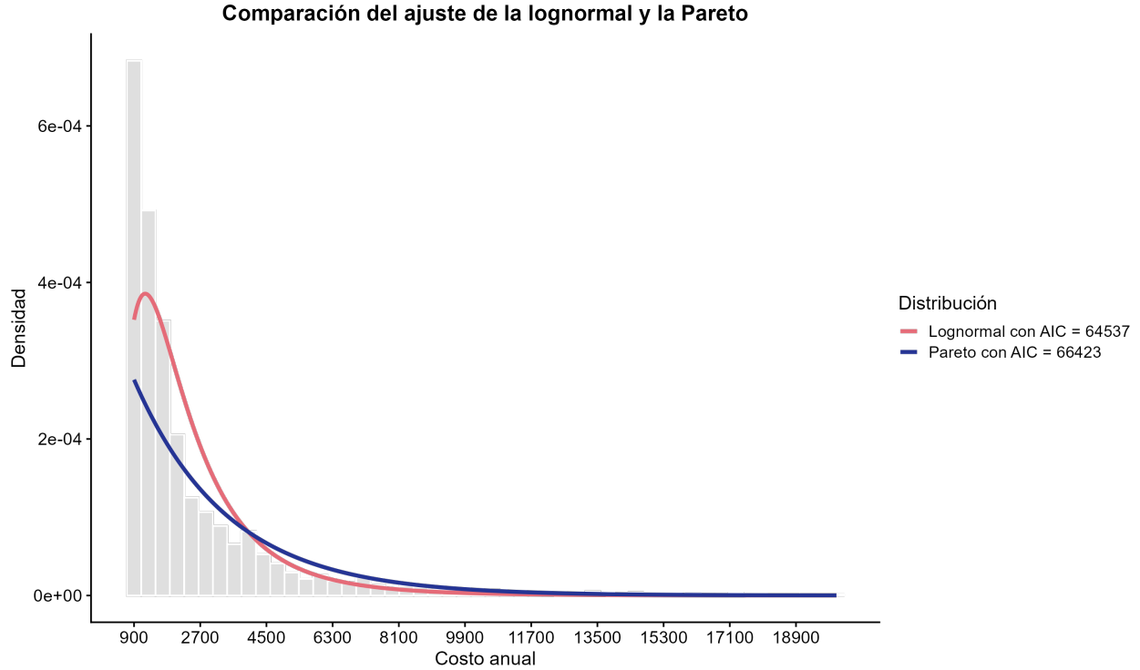
Figura 26: Comparación de las distribuciones Lognormal y Pareto para el intervalo 900 \leq Y \leq 20,000
