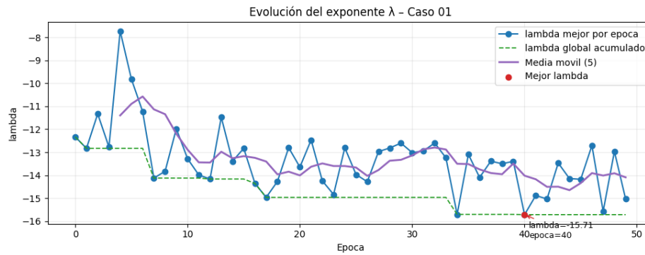
Figura 8.8: Evolución del exponente de Lyapunov por época.
