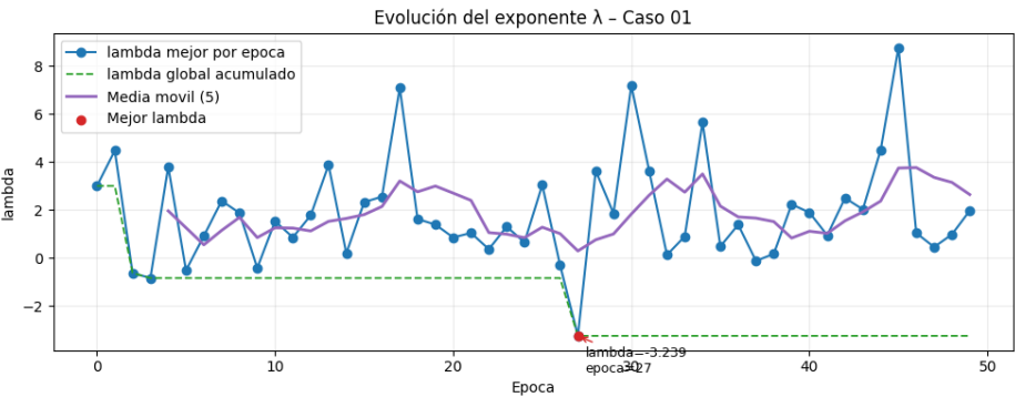
Figura 8.1: Evolución del exponente de Lyapunov por época.
