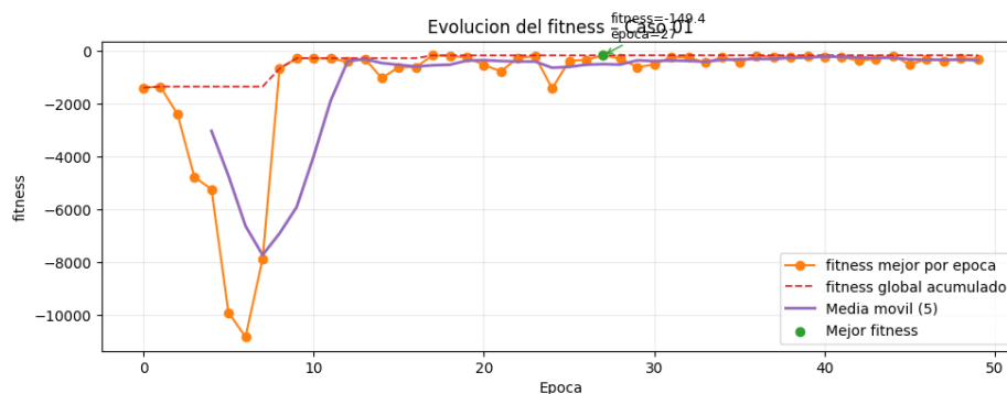
Figura 8.2: Historial del fitness máximo registrado.
