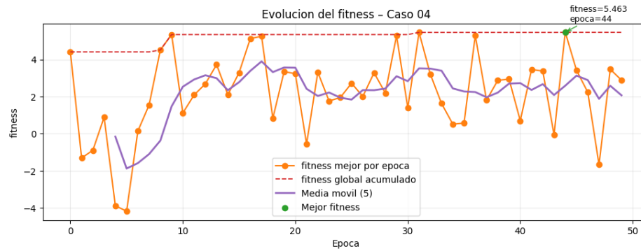
Figura 8.21: Historial del fitness máximo alcanzado en cada época.
