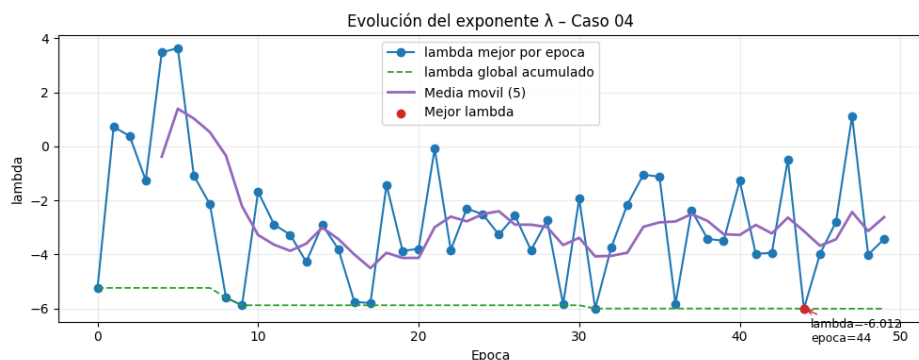
Figura 8.20: Evolución del exponente de Lyapunov para el Caso 04.
