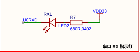
串口 RX 指示灯
