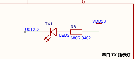
串口 TX 指示灯
