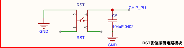
RST复位按键电路模块
