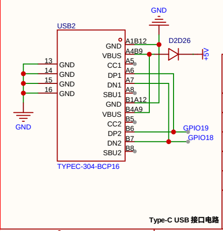
Type-C USB 接口电路
