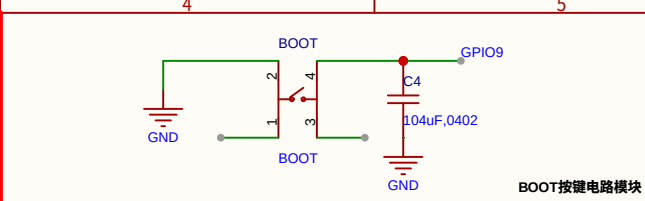
BOOT按键电路模块
