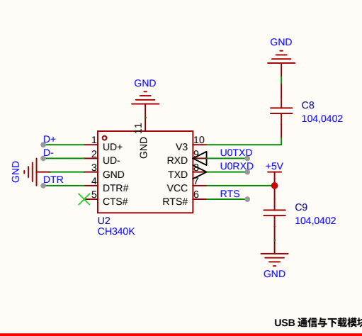
USB 通信与下载模块
