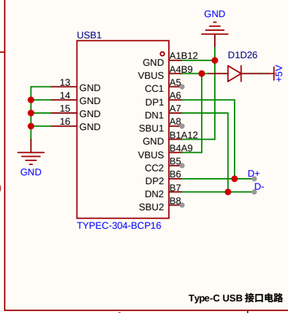
Type-C USB 接口电路
