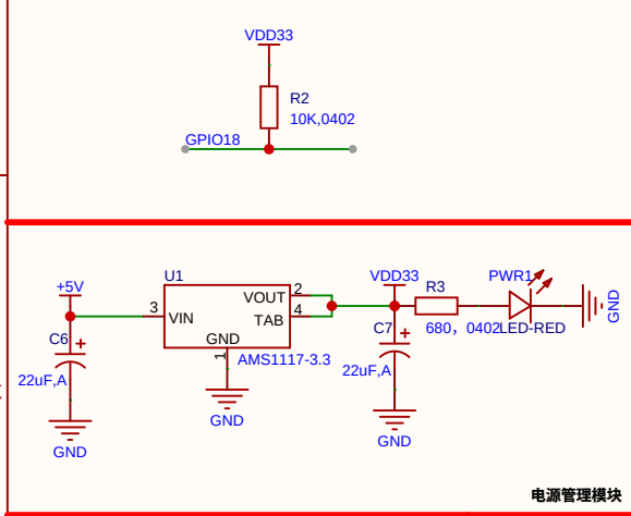
电源管理模块
